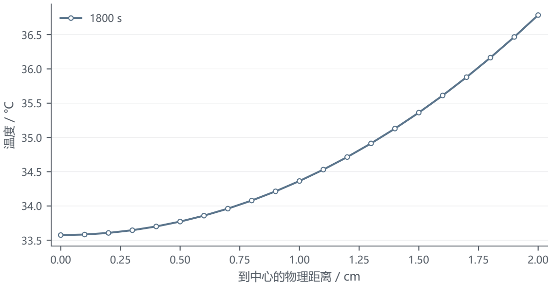
预热末端温度
