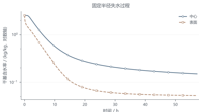
图 4 问题 2-3 固定半径下中心和表面含水率过程。纵轴采用对数尺度以显示后期低含水率层。
