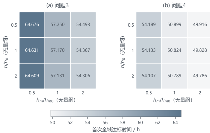
图 10 换热系数和传质系数的 3 \times 3 情景扫描。格内为烘干时长 (h)，所有情景采用同一 161 节点网格和终点规则。
