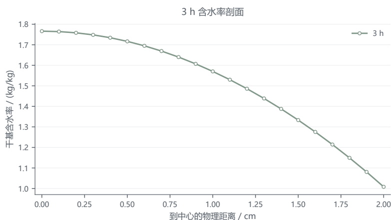
图 5 问题 2 在 3 小时的径向干基含水率结果。
