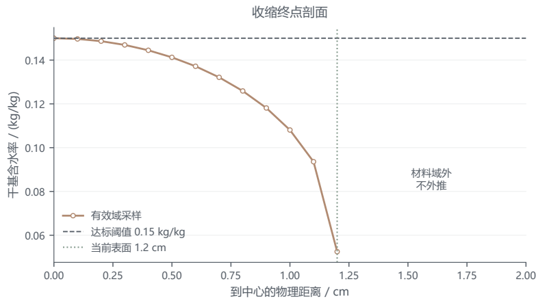
图 9 问题 4 首次全域达标时的固定物理距离含水率剖面；有效域外不进行外推。
