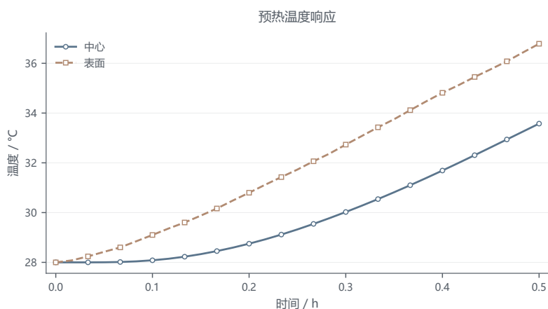
图 2 问题 1 预热阶段中心和表面温度。表面响应快于中心。
