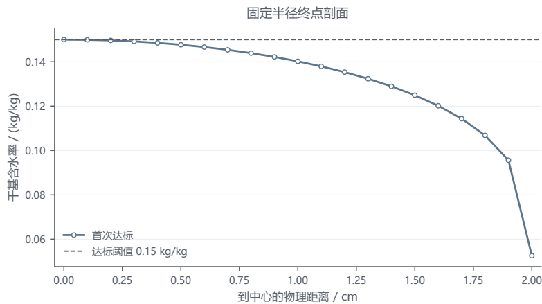
图 7 问题 3 首次全域达标时的径向含水率；虚线为 0.15 阈值。
