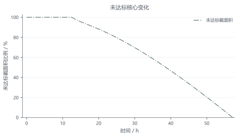
图 6 问题 3 未达标截面积比例随时间变化。
