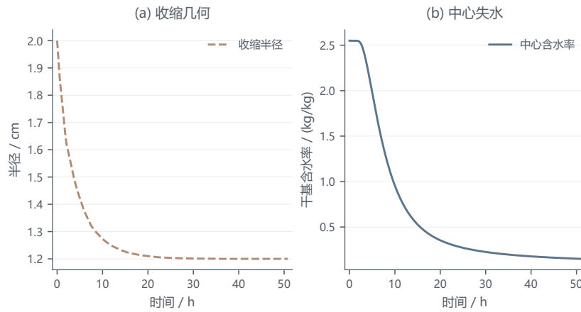
图 8 问题 4 收缩半径与中心含水率的同步变化，采用分面避免双纵轴造成的比较误导。
