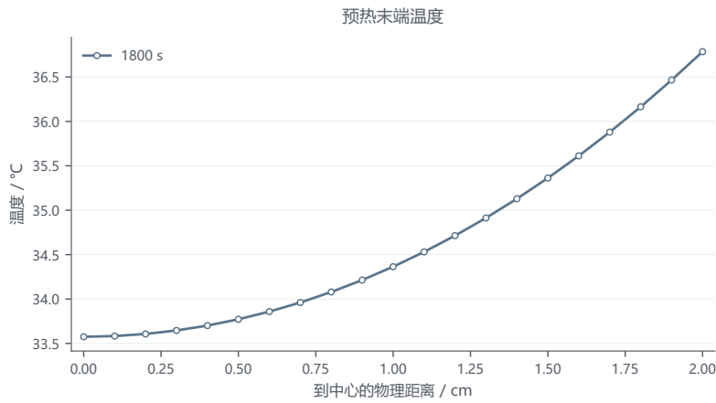
图 3 问题 1 在 1800 秒的径向温度结果。
