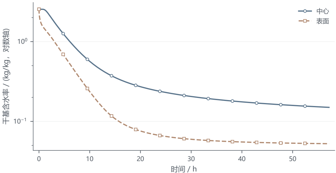
固定半径失水过程
