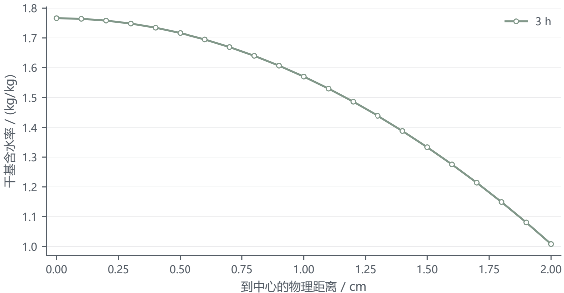
3 h 含水率剖面
