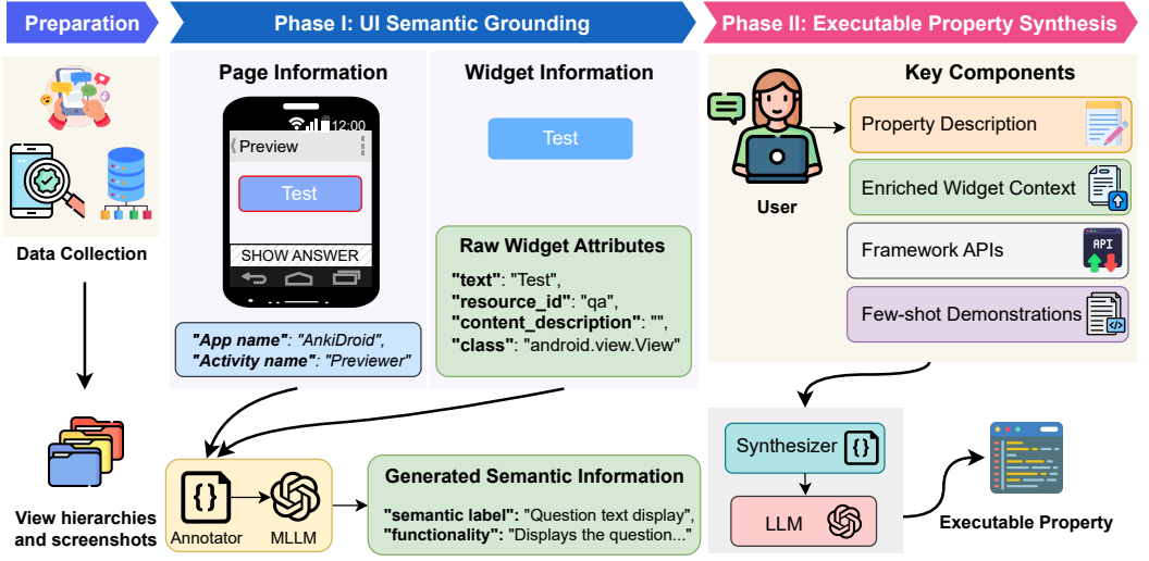
Fig. 2. Overview of iPBT.
