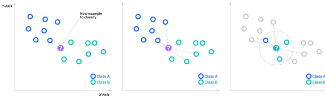
Minh họa thuật toán KNN
