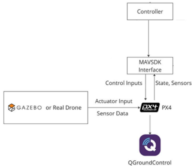
Hình 3. Sơ đồ khối hệ thống
