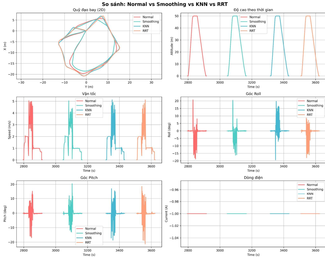
Biểu đồ so sánh tổng hợp 4 phương pháp hoạch định đường bay đã đề xuất
