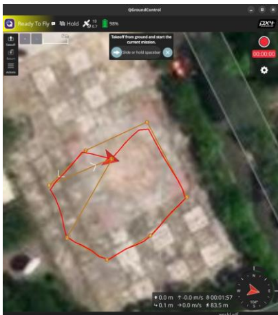
KNN
