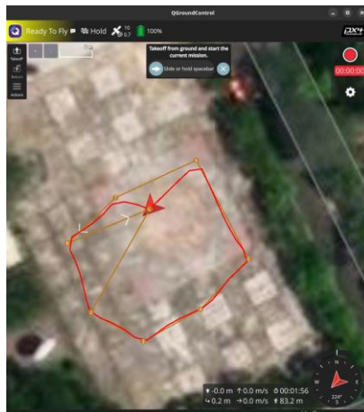
RRT*
