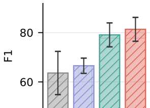
Baron (pancreas)
