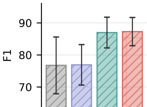
Muraro (pancreas)
