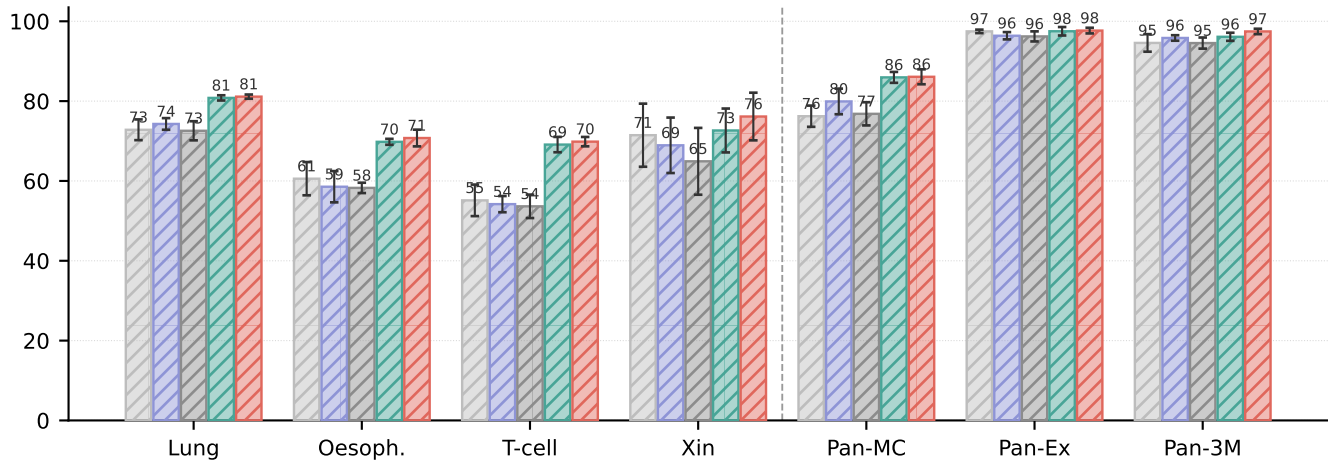
macro-F1
