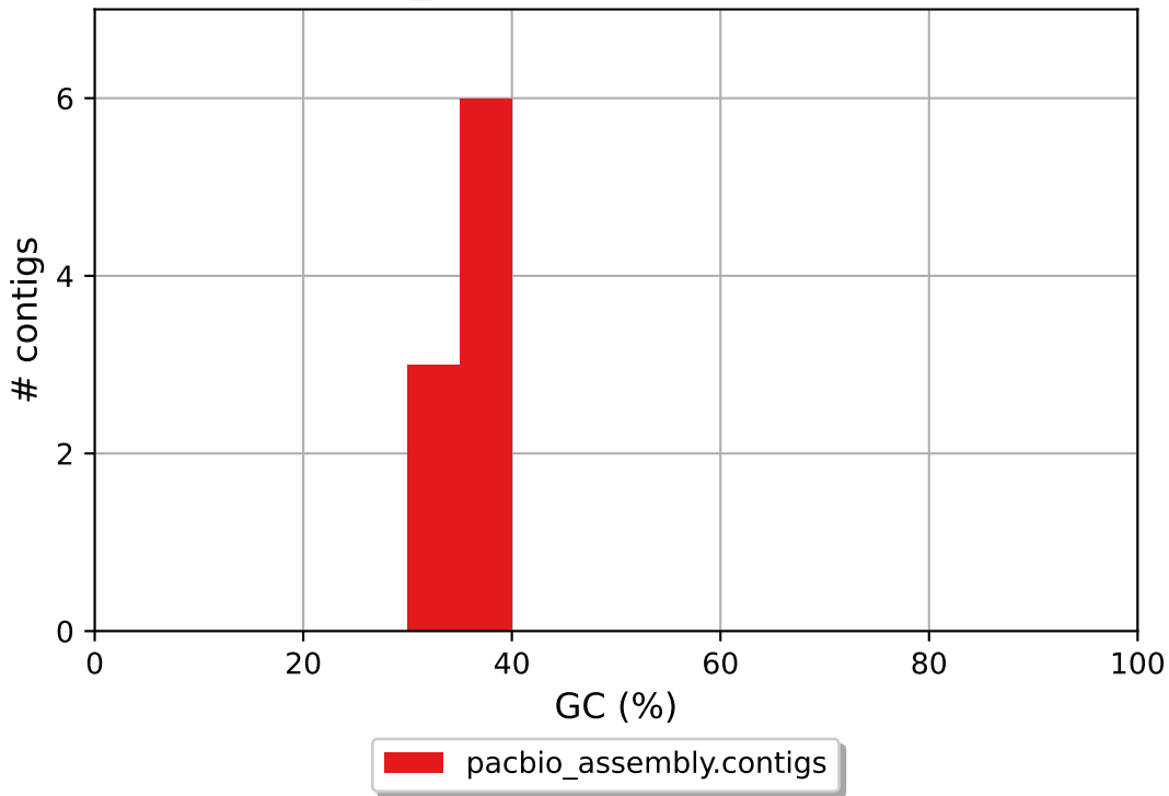
pacbio_assembly.contigs GC content
