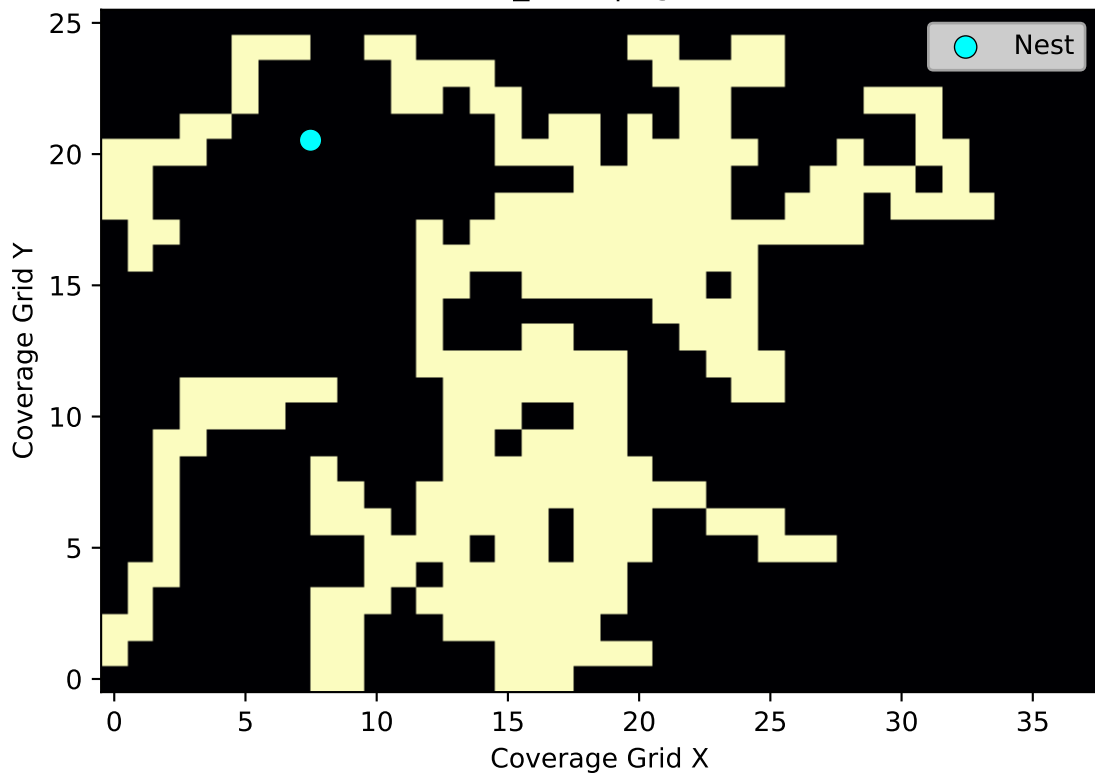
random_walk | agents=10
