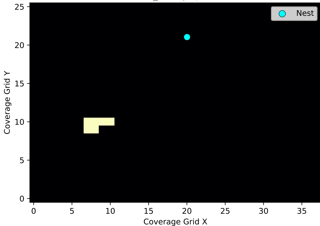
random_walk | agents=1
