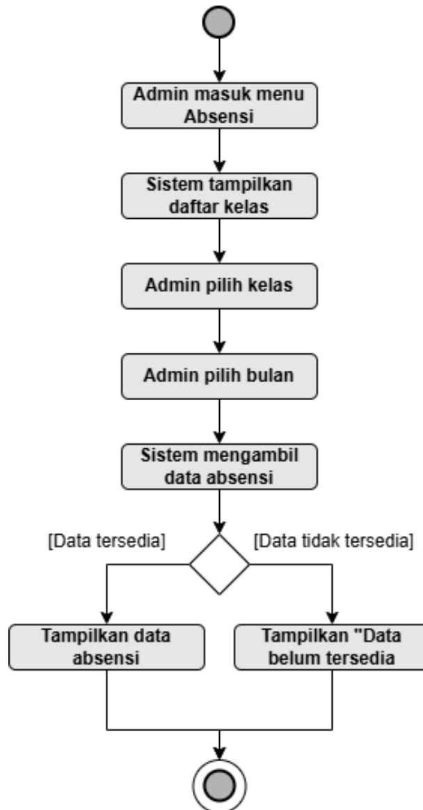
Gambar 3.8. Activity Diagram Melihat Data Absensi
