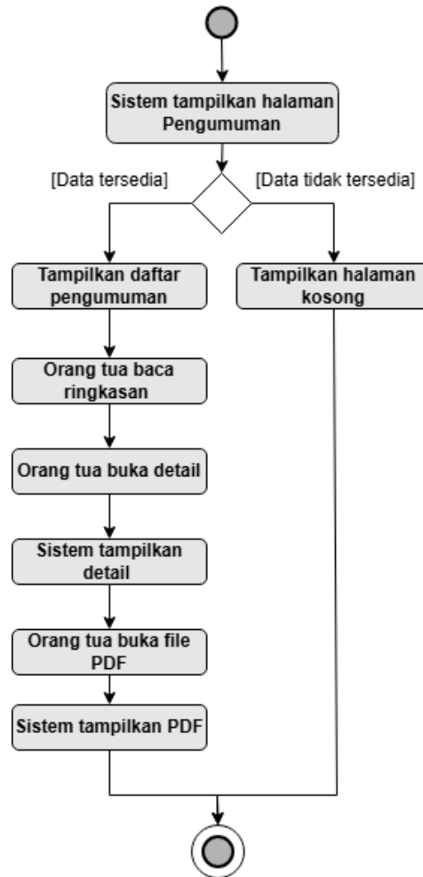
Gambar 3.17. Activity Diagram Melihat Pengumuman
