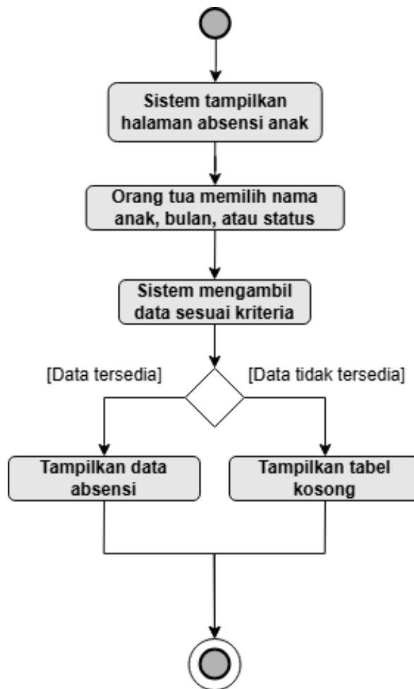
Gambar 3.15. Activity Diagram Melihat Data Absensi
