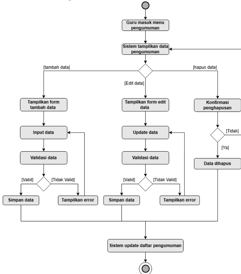
Gambar 3.19. Activity Diagram Kelola Pengumuman
