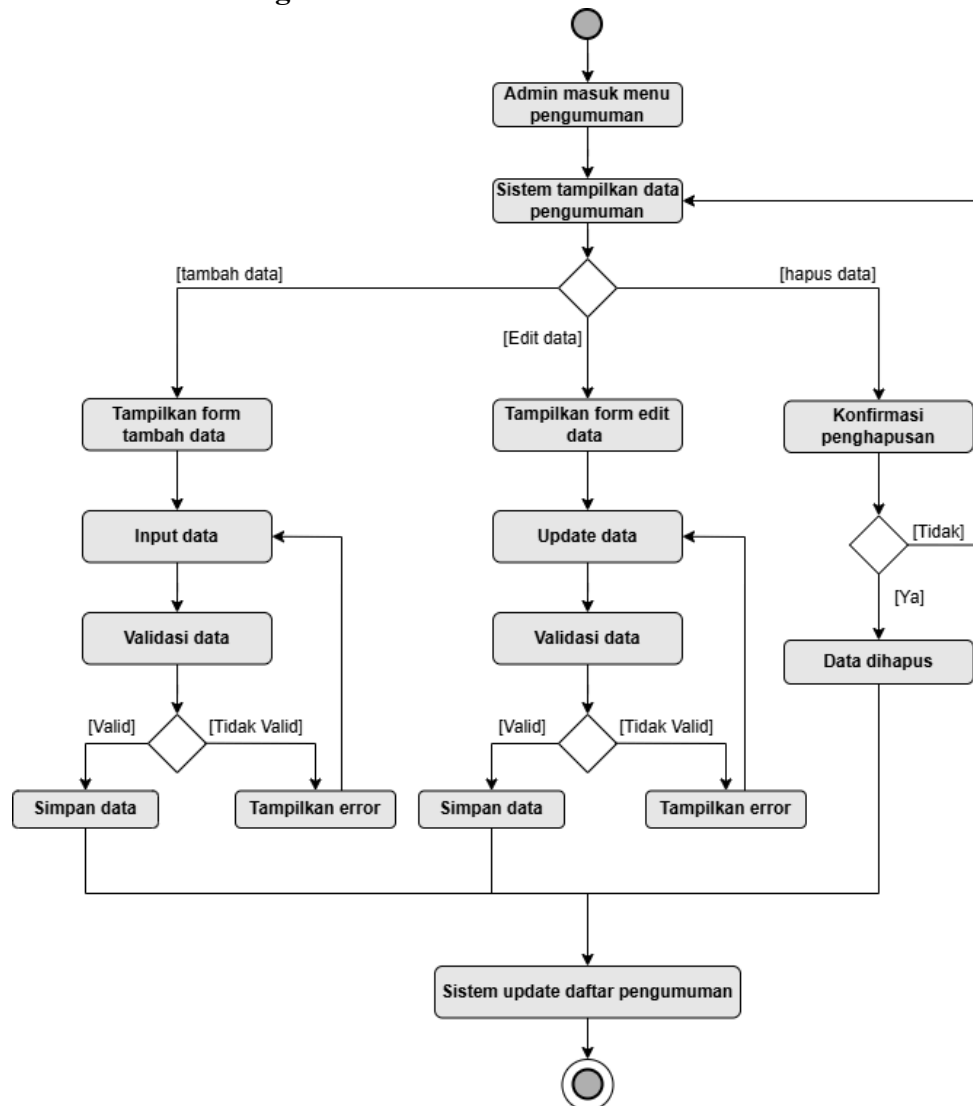
Gambar 3.7. Activity Diagram Kelola Pengumuman
