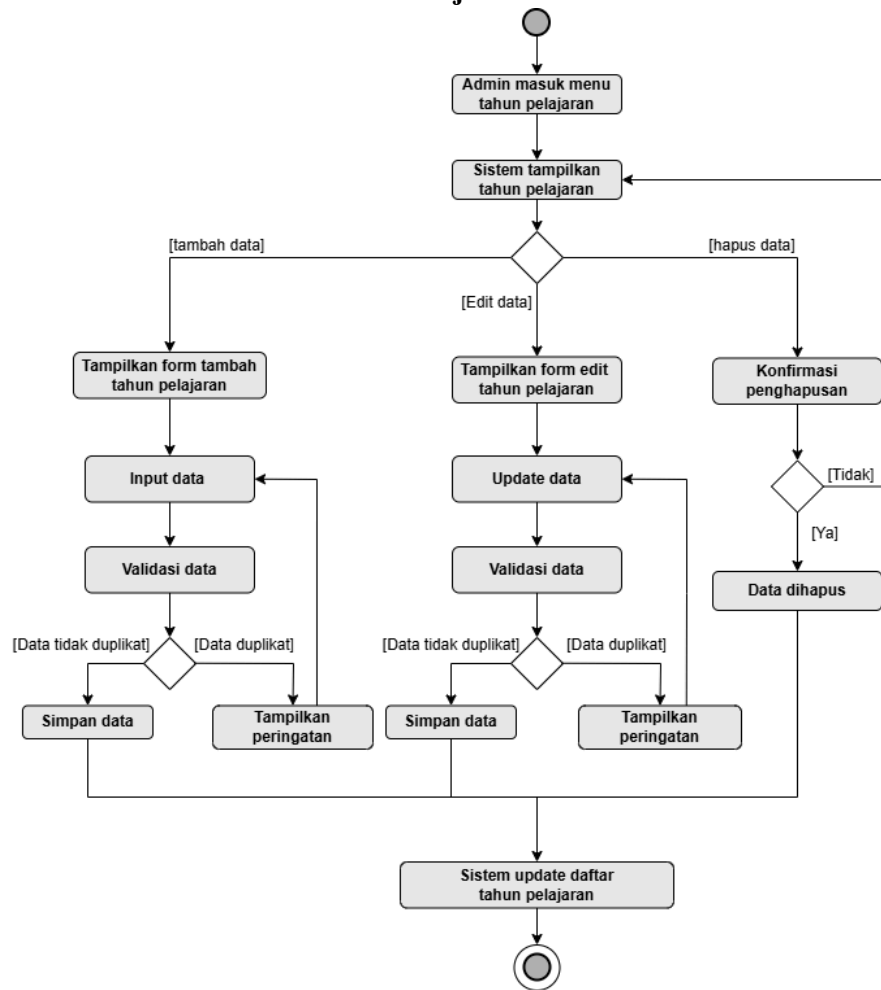
Gambar 3.13. Activity Diagram Kelola Tahun Pelajaran
