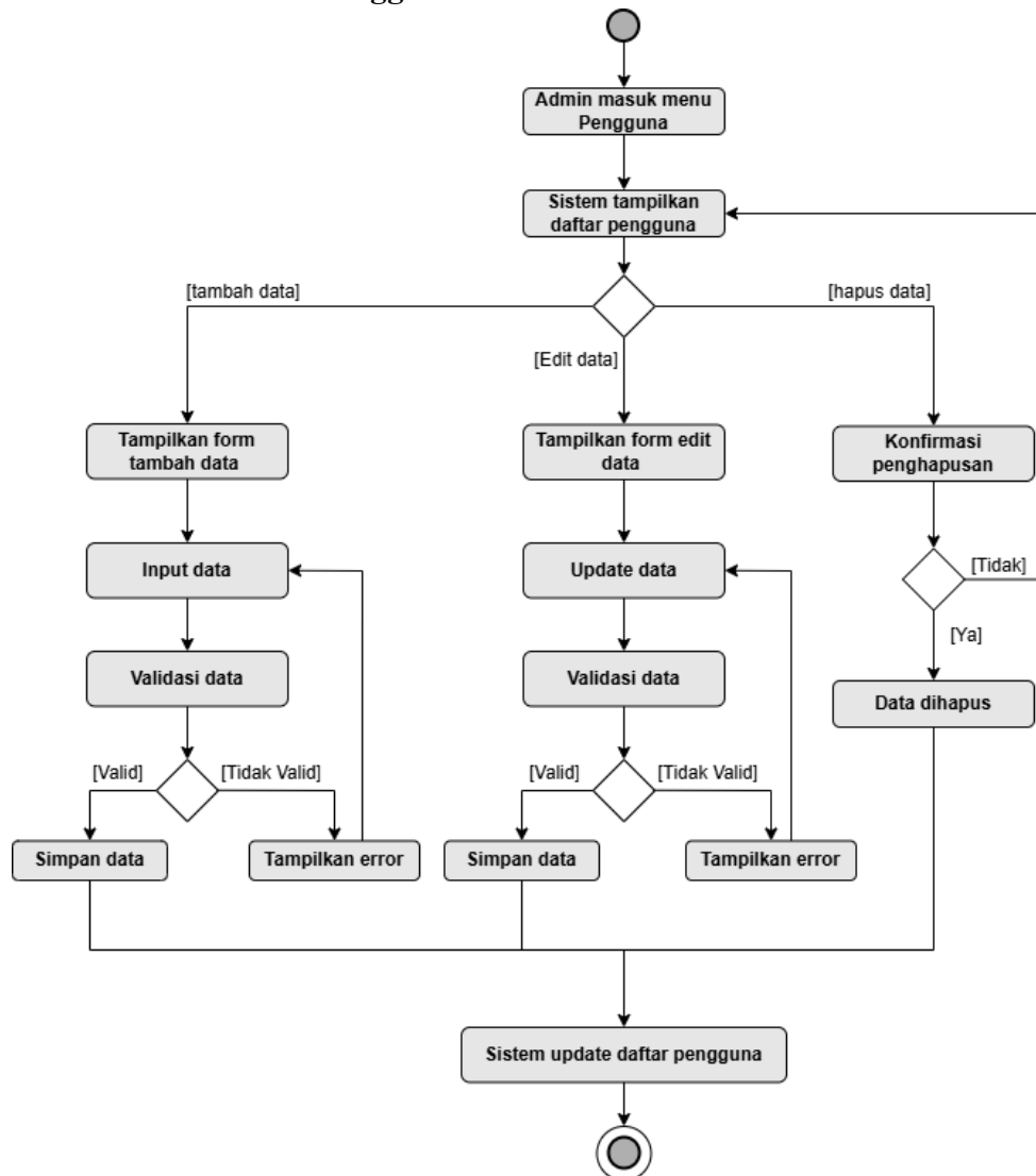
Gambar 3.4. Activity Diagram Kelola Data Pengguna
