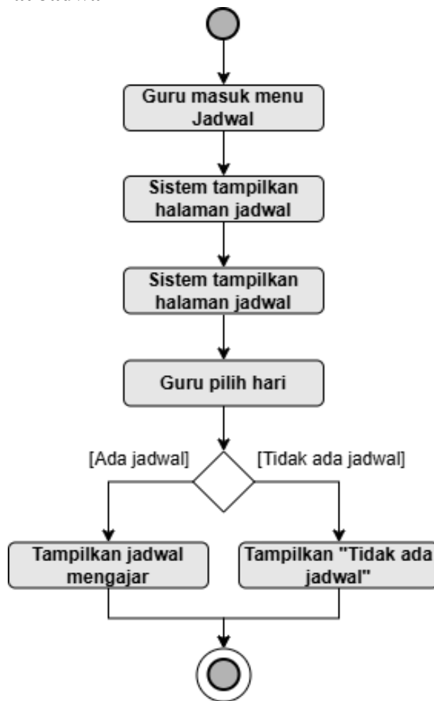
Gambar 3.20. Activity Diagram Melihat Jadwal
