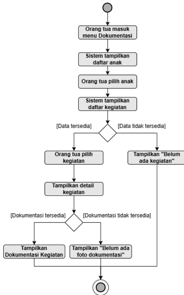
Gambar 3.16. Activity Diagram Melihat Dokumentasi Kegiatan
