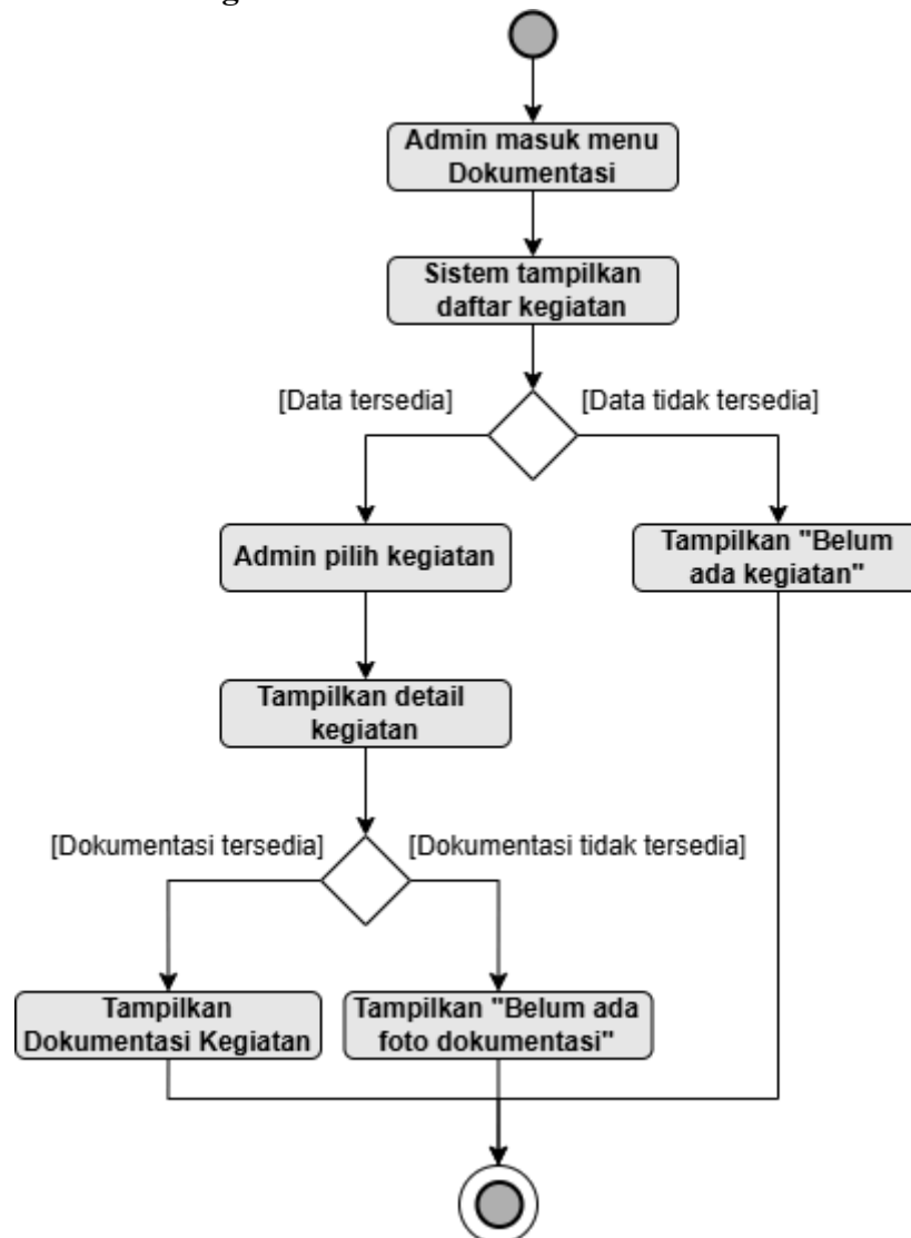
Gambar 3.9. Activity Diagram Melihat Kegiatan dan Dokumentasi
