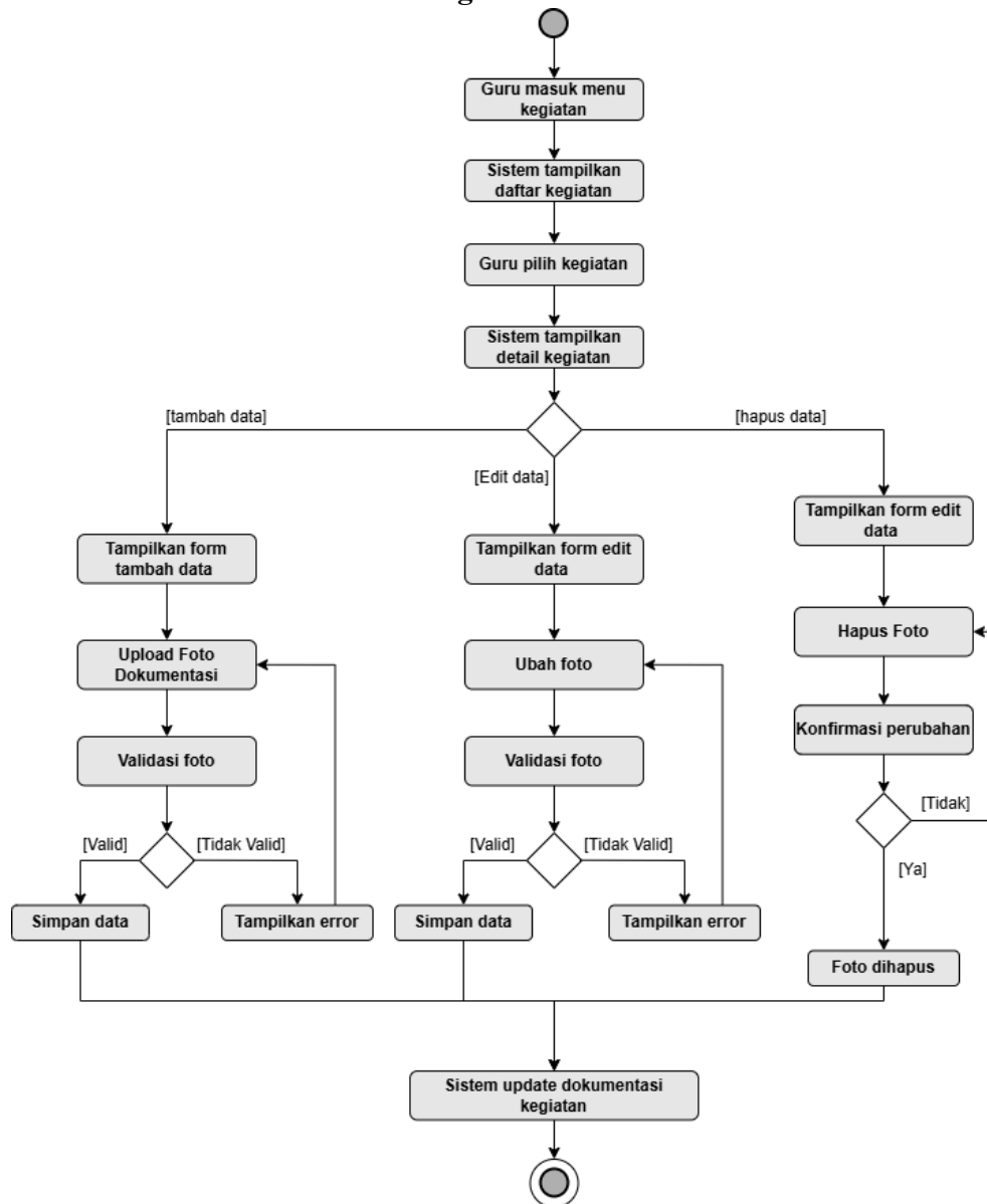
Gambar 3.23. Activity Diagram Kelola Dokumentasi Kegiatan
