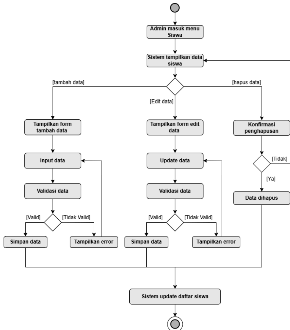
Gambar 3.5. Activity Diagram Kelola Data Siswa
