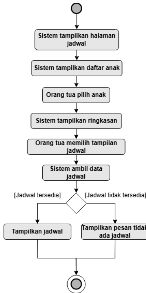
Gambar 3.18. Activity Diagram Melihat Jadwal
