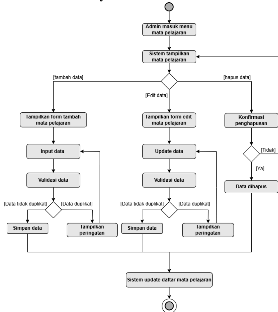
Gambar 3.11. Activity Diagram Kelola Mata Pelajaran
