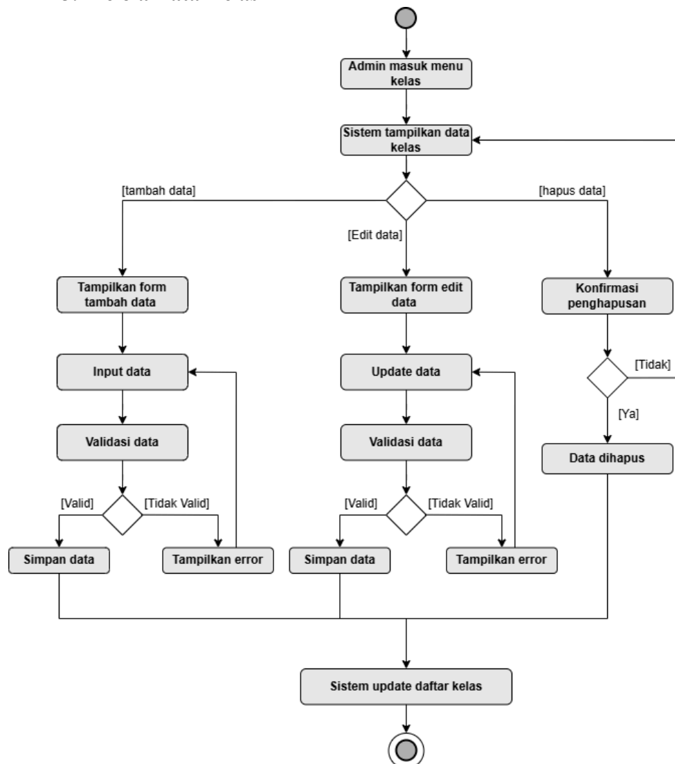
Gambar 3.6. Activity Diagram Kelola Data Kelas
