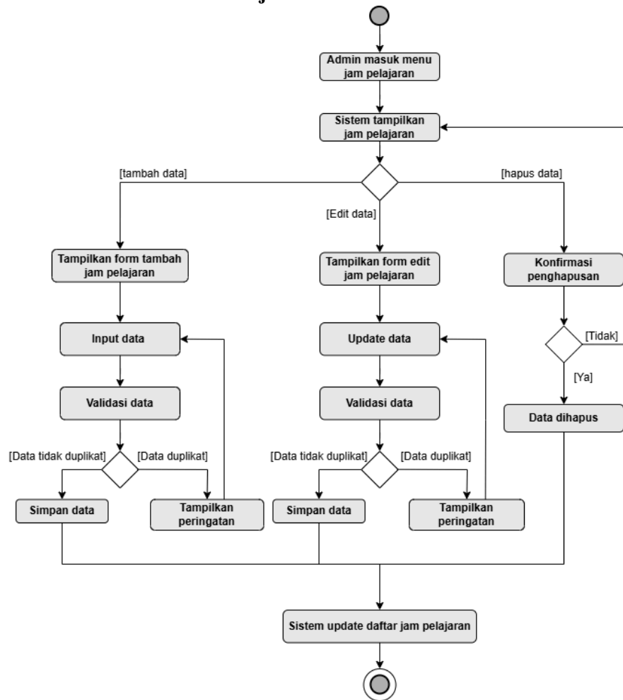
Gambar 3.12. Activity Diagram Kelola Jam Pelajaran
