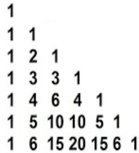
FIGURE 1 – premières lignes du triangle de Pascal
