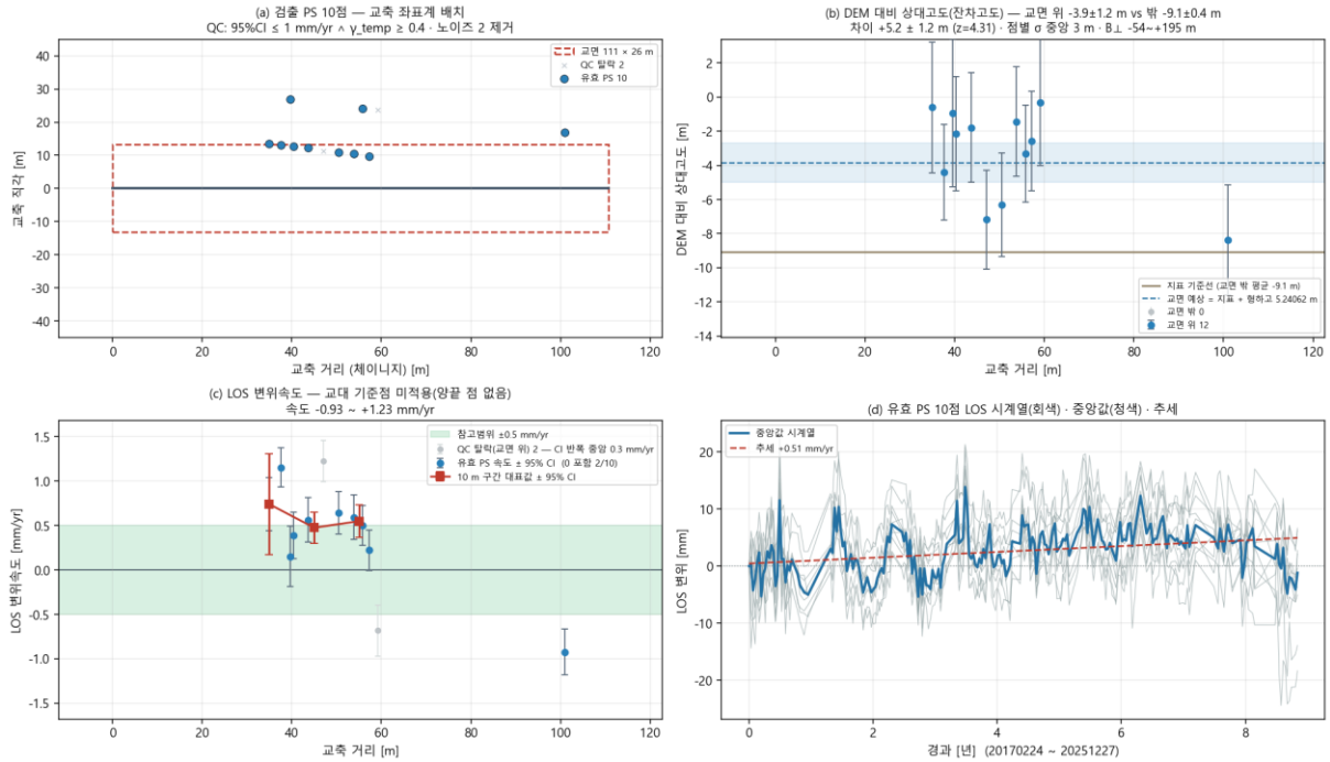
그림 7. brief.png — (a) PS 배치 (b) 잔차고도 (c) 속도 \pm 95% CI (d) 시계열.
