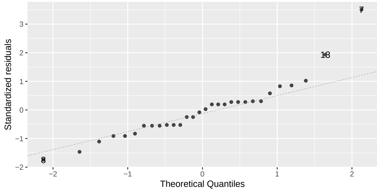
Normal Q-Q
