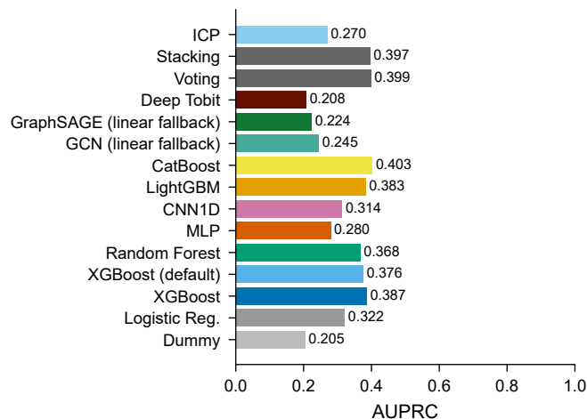
T4 AUPRC
