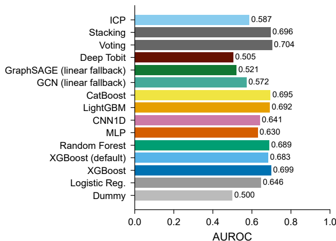
T4 AUROC
