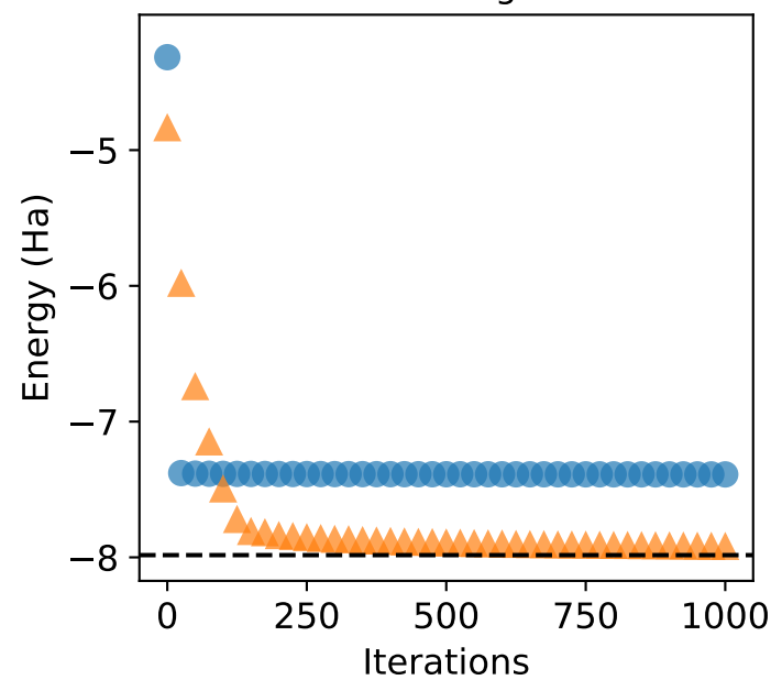
Error scaling: 0.1
