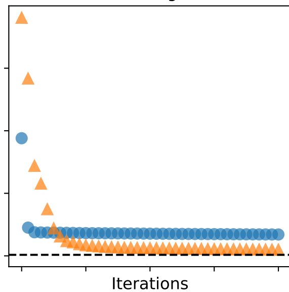
Error scaling: 0.05
