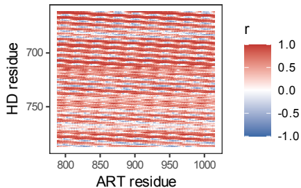
Niraparib
