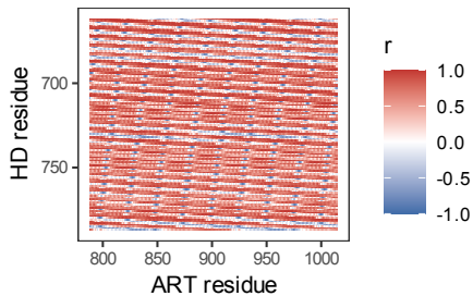
AZD5305
