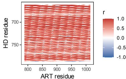
Rucaparib
