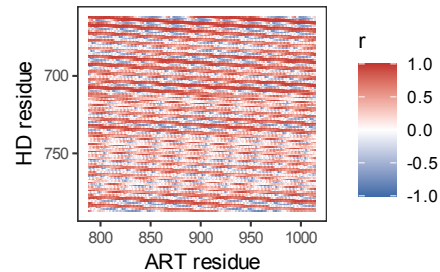
Veliparib
