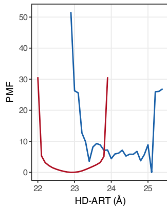
Niraparib
