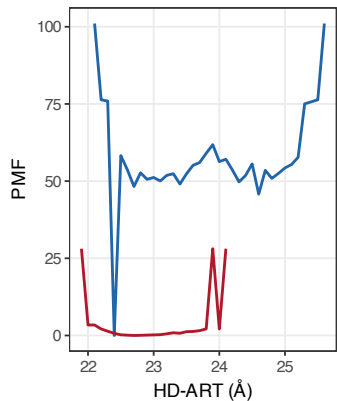
Veliparib
