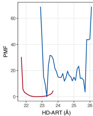
Rucaparib
