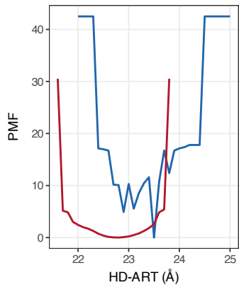
Veliparib
