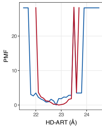
Niraparib
