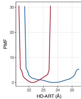
Talazoparib
