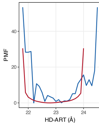
Rucaparib
