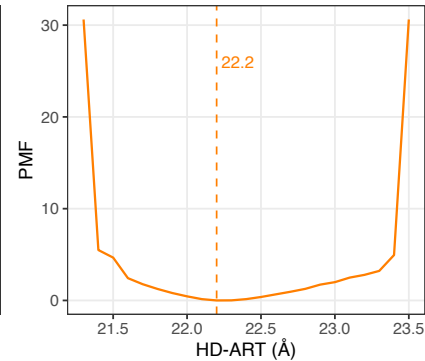
Talazoparib
