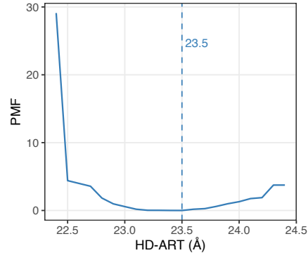
Veliparib
