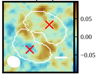
HF(1-0)
