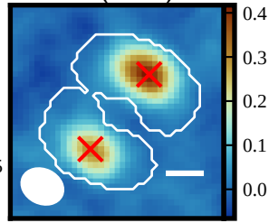
CO(10-9)
