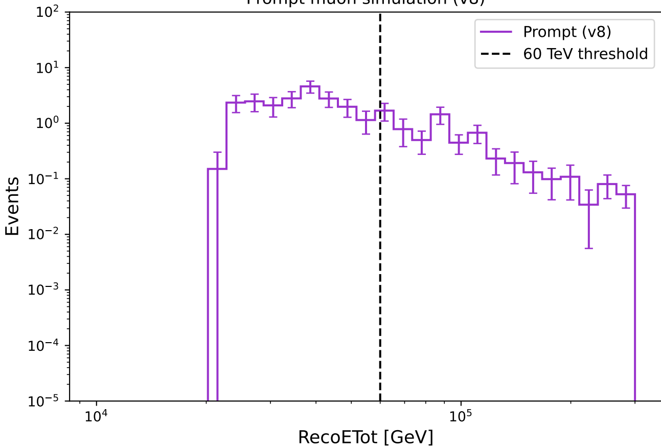
Prompt muon simulation (v8)
