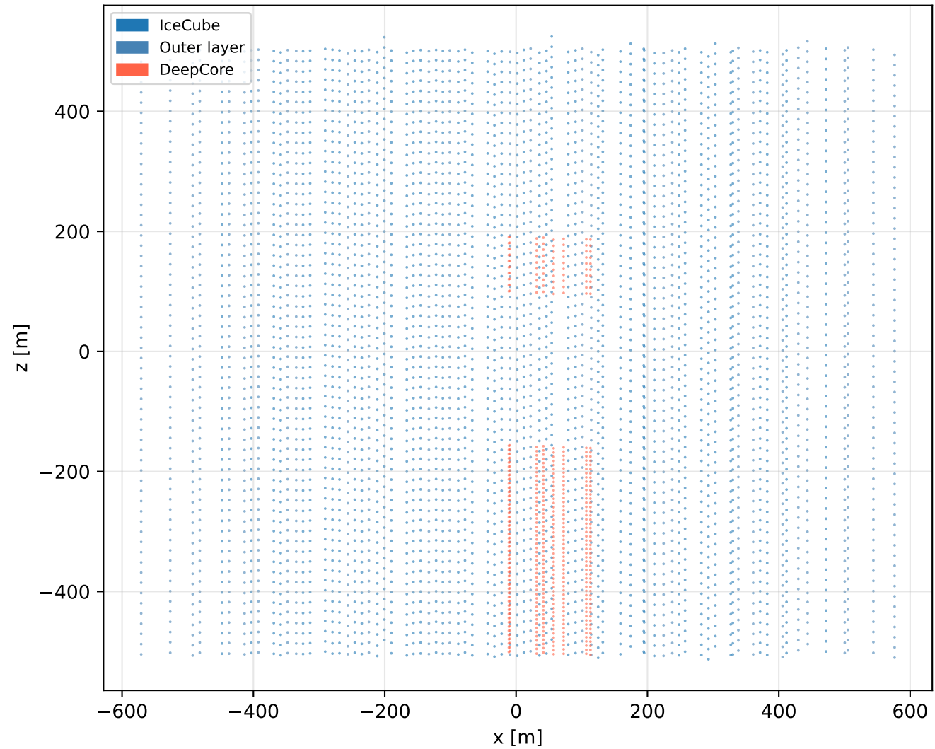
Side view (ZX)
