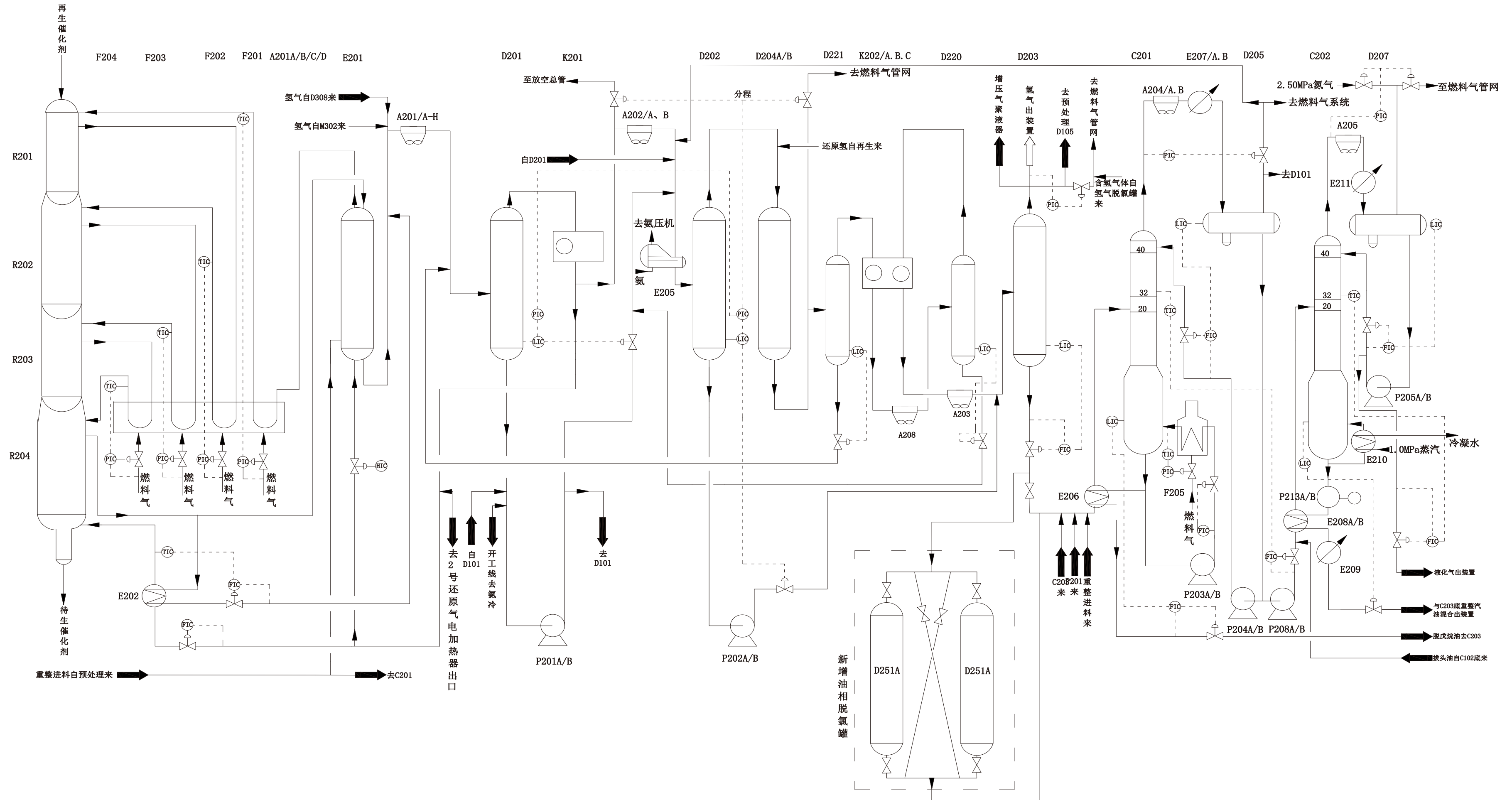
延安石化厂120万吨/年连续重整反应部分工艺流程图
