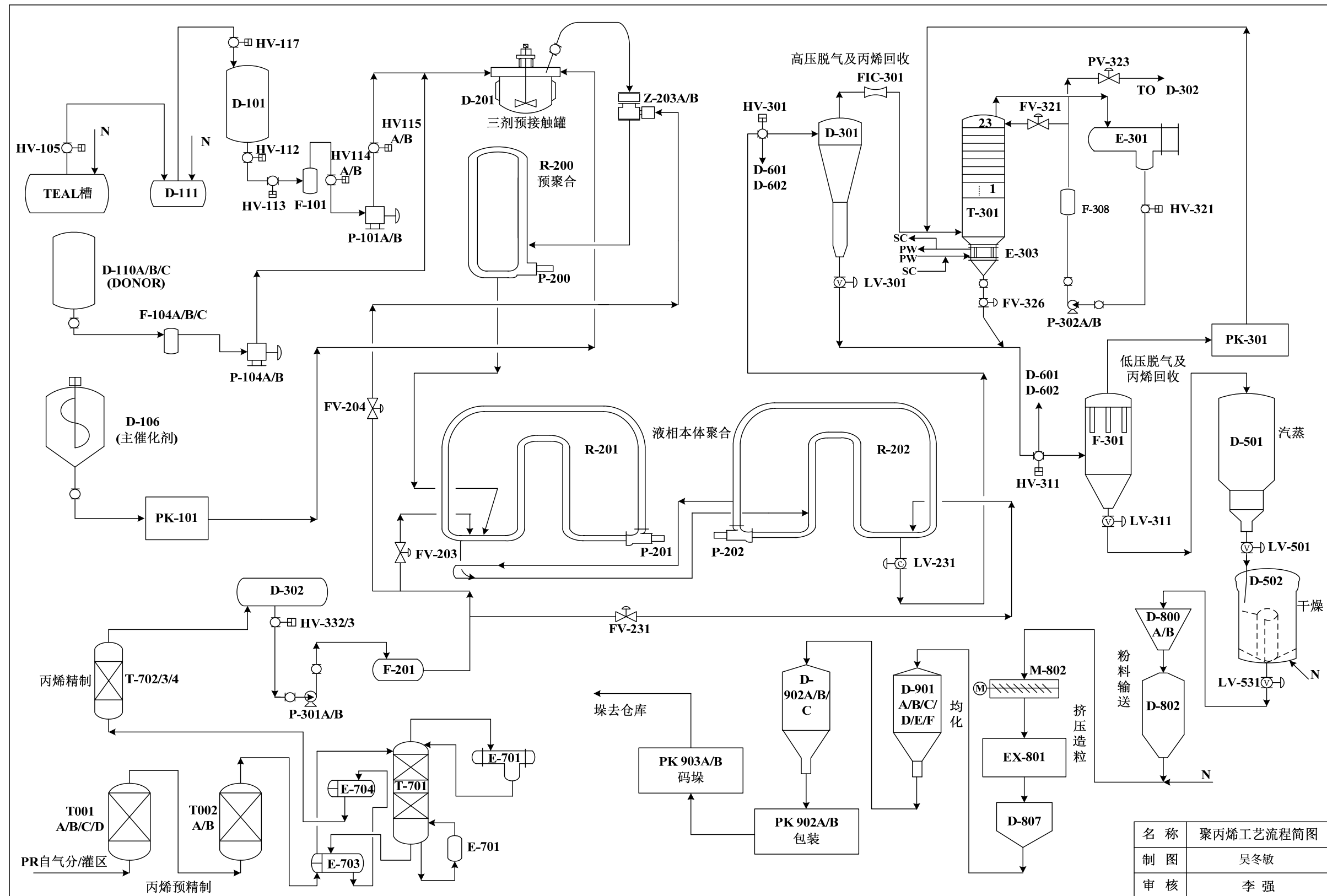
20wt/a 聚丙烯工艺流程简图
