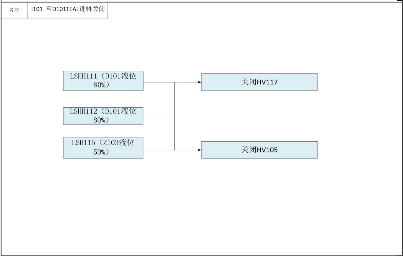
附件六 《20万吨/年聚丙烯装置联锁逻辑示意图》
