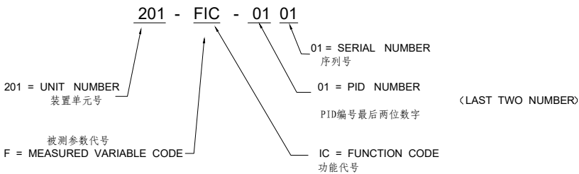
INSTRUMENT NUMBERING 仪表编号
