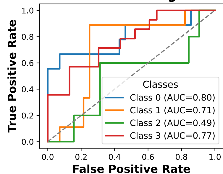
GradientBoosting ROC
