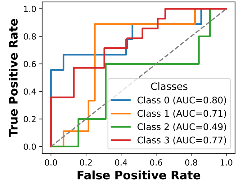
GradientBoosting ROC (ROS + IQR)
