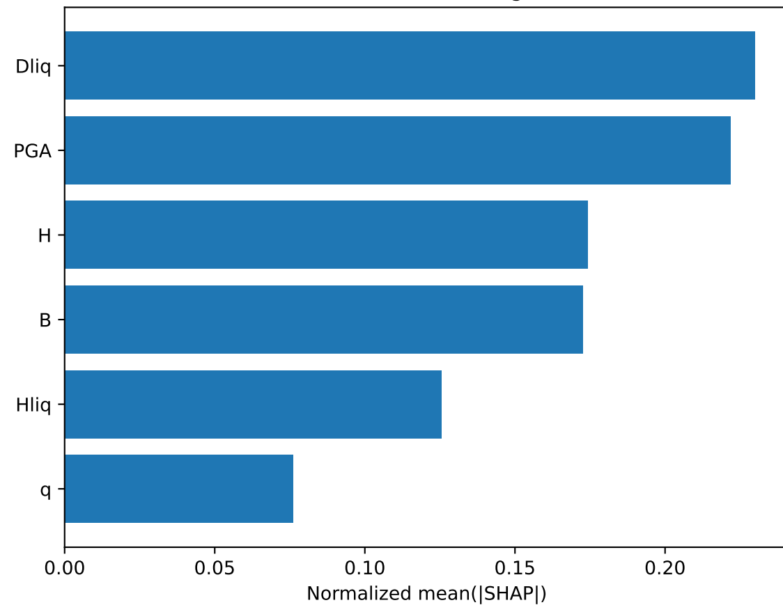
GradientBoosting
