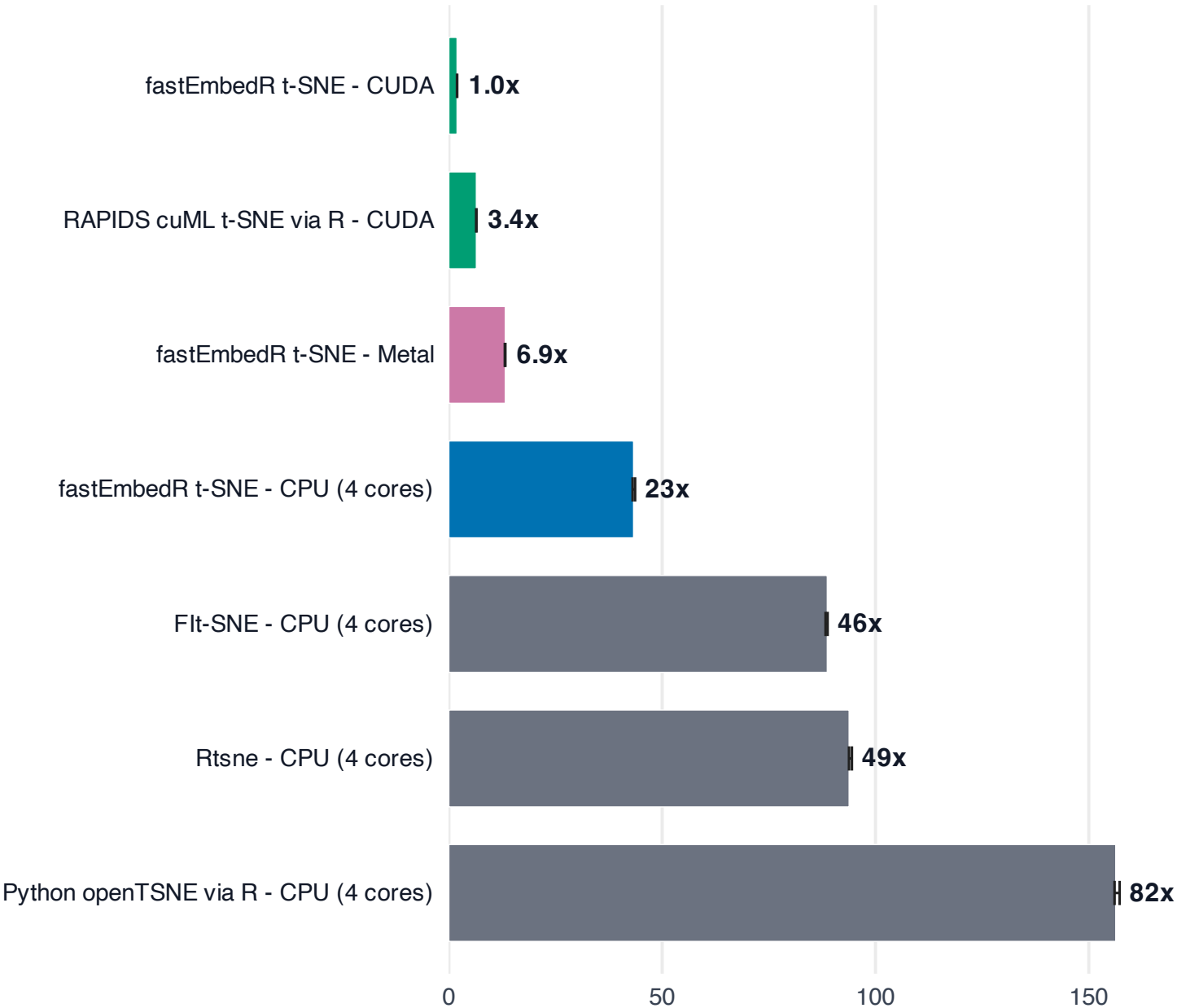
t-SNE
