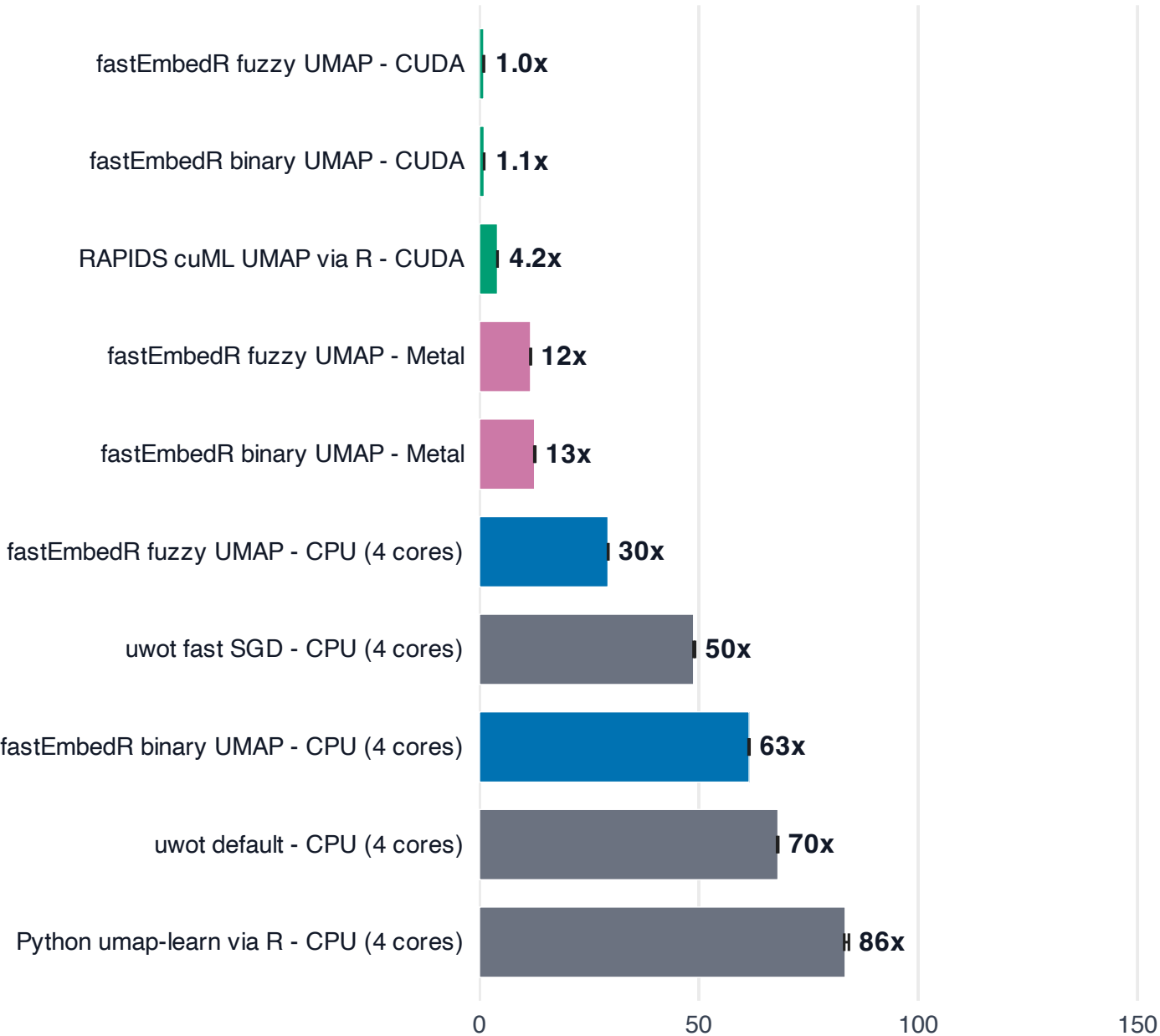
UMAP
