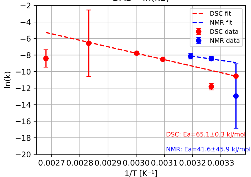
DAB - ln(k1)
