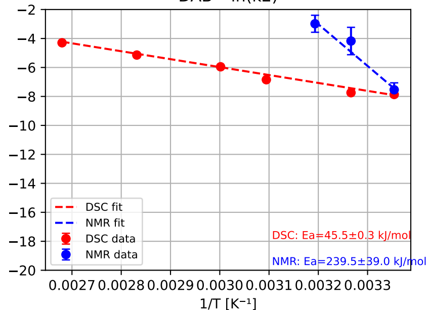
DAB - ln(k2)
