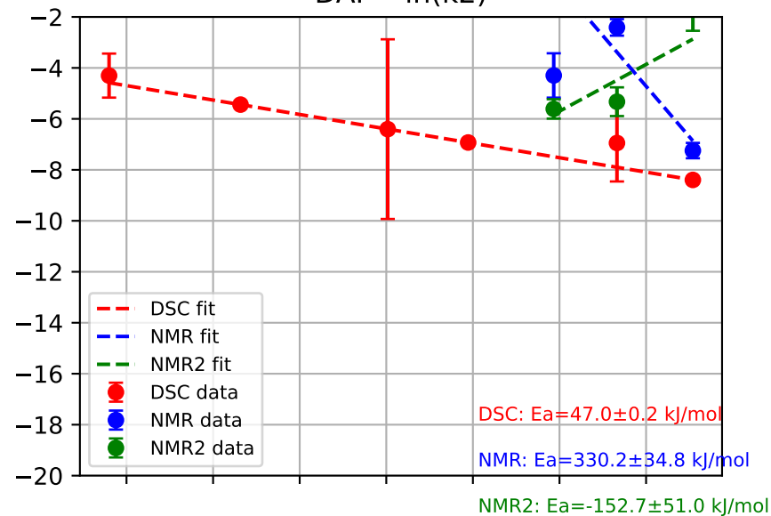
DAB - ln(k2)
