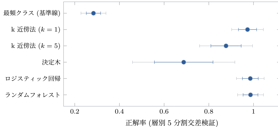
図 8.7 6 手法のフォレストプロット。点が層別 5 分割交差検証の平均正解率、濃い細い棒がその手法だけを見たときの 95% 信頼区間、薄い太い棒が 6 手法をまとめて 95% にした区間である。表を眺めるより、どの差が読み取れてどの差が読み取れないかが早く分かる。区間はいずれもフォールド間の SD/\sqrt{5} を標準誤差とした t 区間で、フォールドが独立でないため (第 8.3.4 項)、正式に 95% の被覆を保証する区間ではない。描き方の説明用と考えてほしい。
