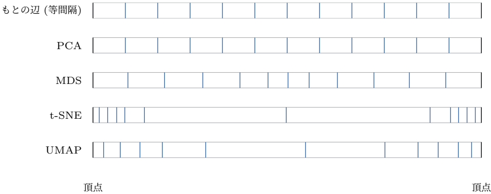
図 6.16 1 本の辺を長さ 1 に伸ばし、13 個の点が来た位置に縦線を引いたもの (192 本の辺の中央値)。両端の太い黒線が頂点。もとは等間隔なので、素直に写っていれば縦線も等間隔に並ぶ。t-SNE では 11 本が両端に張りついて、真ん中が大きく空いている
