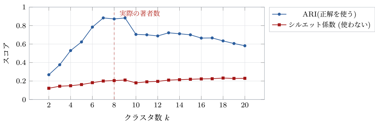
図 5.6 クラスタ数と 2 つの評価指標 (Ward 法)。
