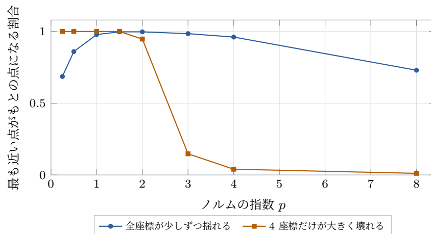
図 4.19 ずれ方の型ごとの、最も近い点の当たり方。次元は両条件とも 100 で、ずれの総量もそろえてある。それでも最適な p が 2 付近から 1 以下まで移る。
