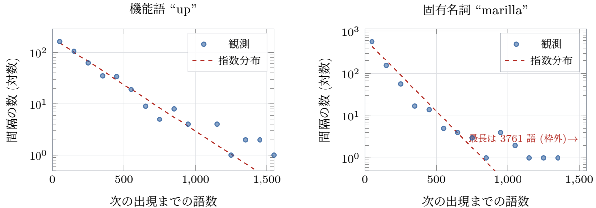
図 2.5 同じ 2 つの単語を「間隔」で見る。縦軸が対数なので、指数分布は直線になる。“up” は乗るが、“marilla” は短い間隔が多すぎ、長い間隔也多すぎる。
