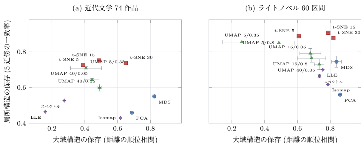
図 6.21 点は乱数の種 5 通りの平均で、誤差棒は縦横それぞれの標準偏差である (横棒が大域構造の指標のばらつき、縦棒が局所構造の指標のばらつき)。縦棒が短いのは、局所の指標が種を変えてもほとんど変わらないためである。右上に行くほど良い。t-SNE に添えた数字は perplexity、UMAP の数字は n_neighbors/min_dist である。UMAP は 9 通り試したうち、他のどの設定にも両軸で負けていない設定だけを細い線で結んで載せた。近代文学では右上の角が空くが、まとまりの強いライトノベルでは t-SNE がそこに近づく。トレードオフの強さはデータで変わる。
