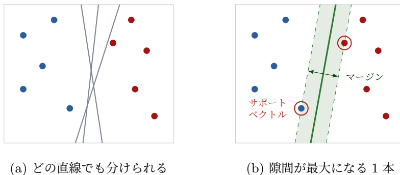
図 7.5 境界の引き方。2枚とも同じ点である。(b)の破線は、境界から左右に等しく離れたマージンの縁で、赤い輪をかけた2点がちょうどその上に乗る。この2点が境界を決めており、これより境界に近い点は存在しない。
