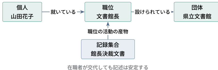
図 4.5 職位 (Position) の使いどころ。記録を「個人」でも「団体」でもなく「職位」に結びつけることで、人事異動に左右されない記述ができる (RiC-E12 スコープノートに基づく)。
