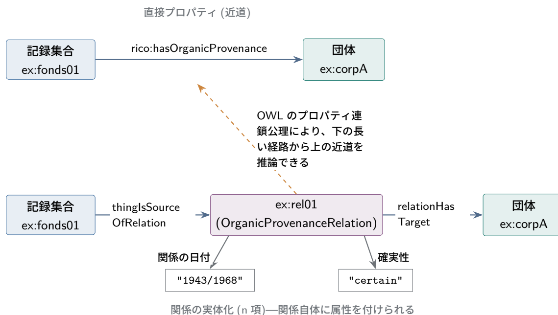
図 5.4 同じ出所関係の 2 つの表現。RiC-O では多くの直接プロパティが「実体化された関係を経由する長い経路の近道」として形式的に定義されており、長い経路を書けば近道は推論で得られる (第 6 章)。
