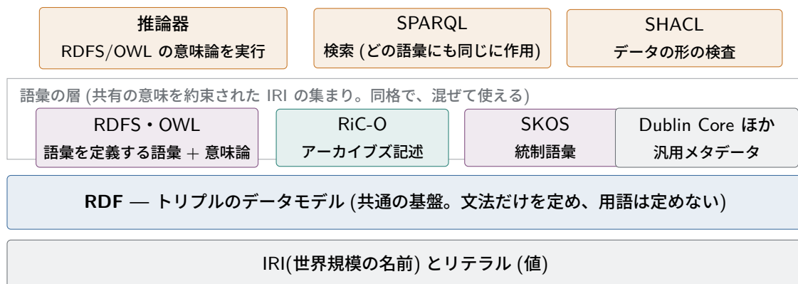
図 5.2 層構造の見取り図。基盤は RDF(トリプル) だけ 1 つで、その上に載る語彙はすべて同格である。RDFS・OWL だけが「語彙を定義し、推論の意味論を与える」という特別な役割を持ち、SPARQL や SHACL はどの語彙のトリプルにも同じに働く。
