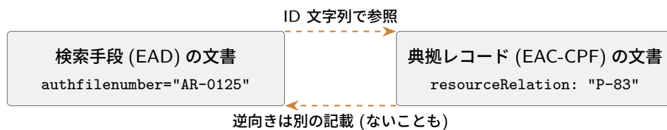
(a) 文書ベース: 参照は文書中の記載。2 本は独立で、同期の保証がない
