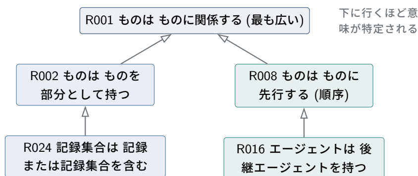
図 4.4 関係のポリヒエラルキー (RiC-CM §5.3 の一部)。狭い関係で記述しても、広い関係としても成立している (第 6 章の推論はこれを利用する)。
