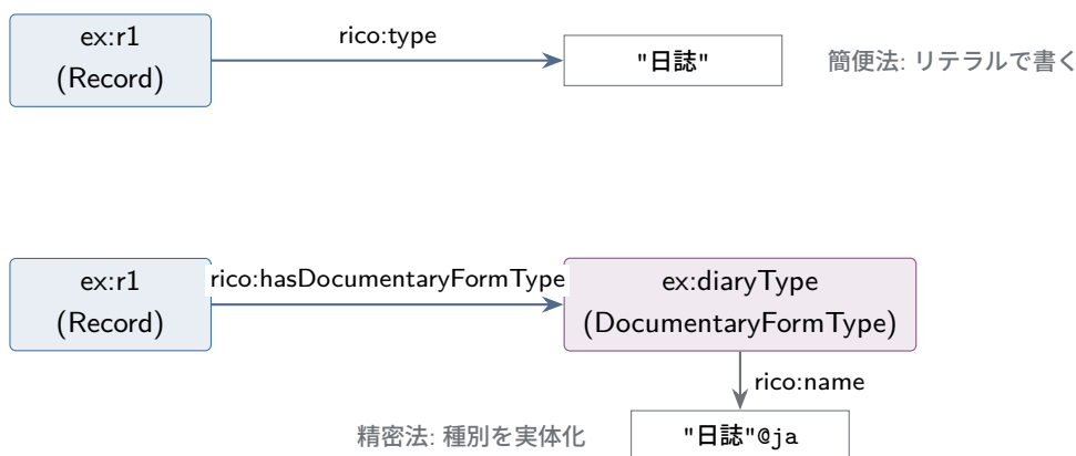
図 5.3 同じ情報の2つの書き方 (上: 簡便法、下: 精密法)。精密法なら種別自体を SKOS 語彙として整備し、多言語ラベルや上位下位関係を持たせ、機関を越えて共有できる。
