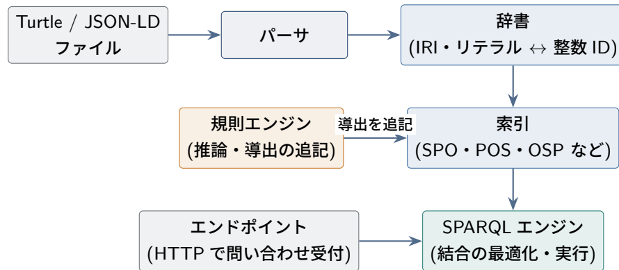
図 6.5 トリプルストアの内部構成のあらまし。RDB でいえば、辞書と索引は B 木索引、SPARQL エンジンは実行計画の最適化器に当たる。
