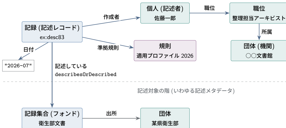
図 4.6 記述の記述の仕組み。目録データそのもの (記述レコード) が一段上の階の記録になり、記述者・規則・日付はその属性・関係として付く。2つの階は rico:describesOrDescribed という通常の関係でつながる。記述者・職位・機関は、記述対象の階の実体とまったく同じクラスである。
