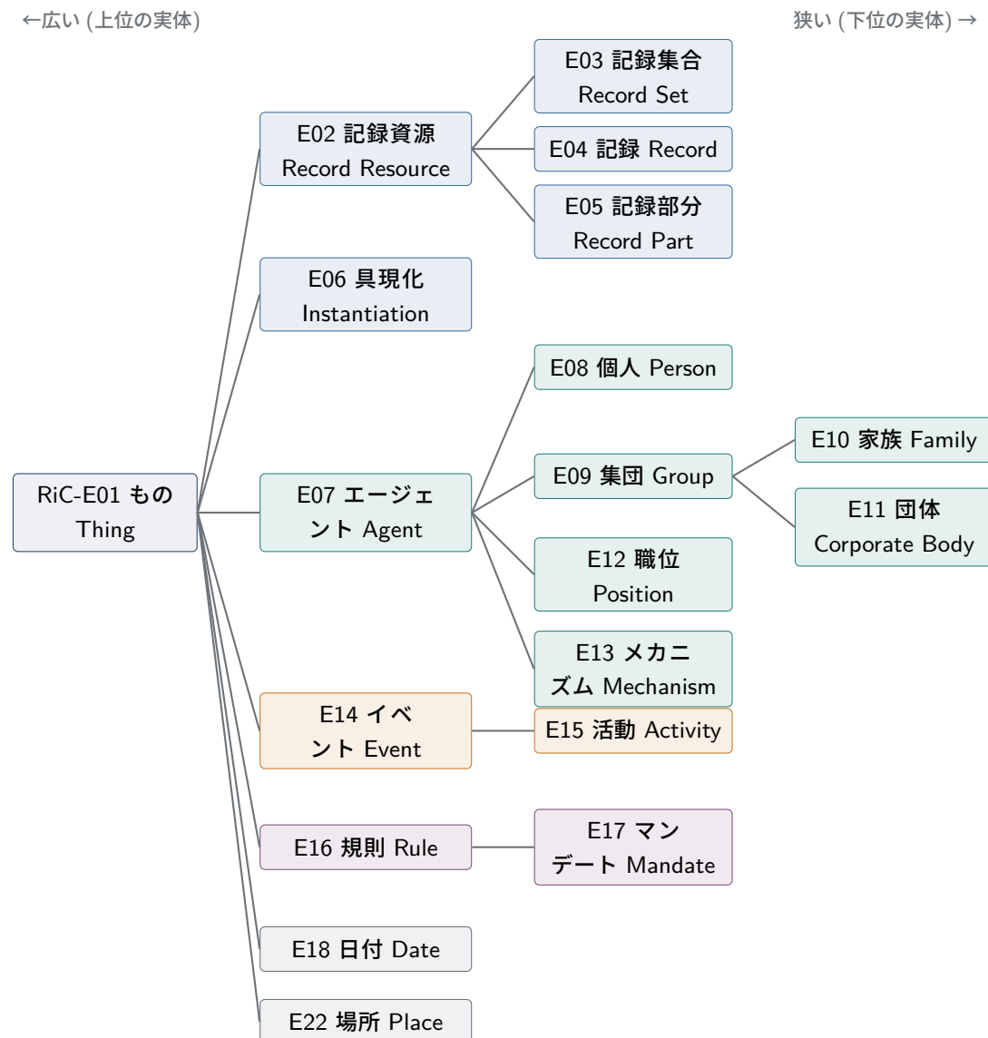
図 4.2 RiC-CM 1.0 の実体階層 (RiC-CM §2.1 の表に基づく)。線はすべて「～の一種である (is a kind of)」を表す。記録集合が記録を「含む」という関係はこの図には現れないことに注意 (§4.4)。E19-E21 が欠番なのは、0.2 版にあった日付の下位実体 (単一日付・日付範囲・日付集合) が 1.0 で廃止されたためである。
