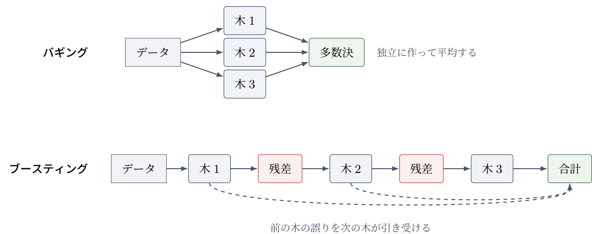
図 7.9 バギングとブースティングの違い。前者は並列、後者は逐次。
