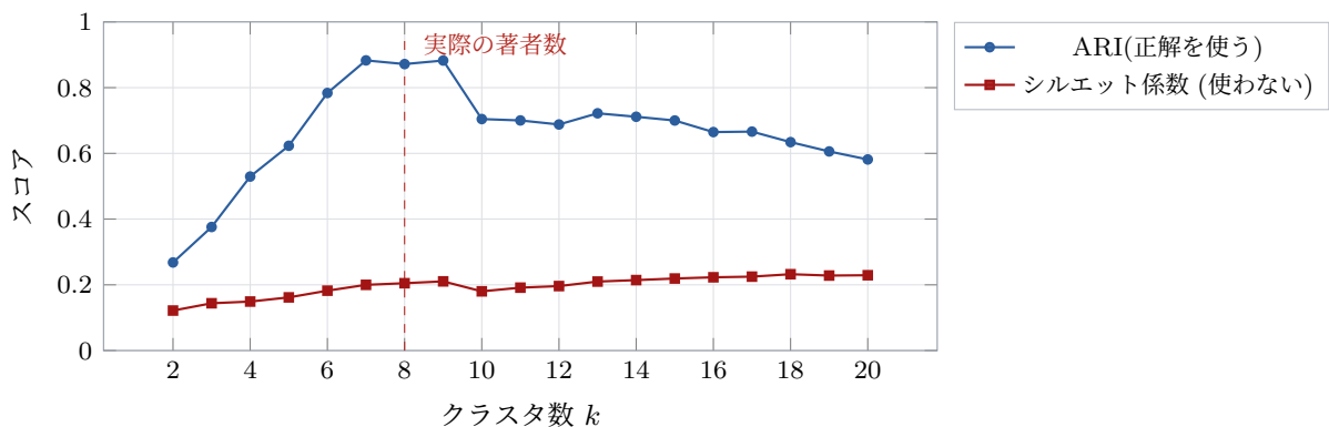
図 5.6 クラスター数と 2 つの評価指標 (Ward 法)。
