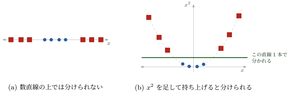
図 7.6 次元を上げると直線で分けられるようになる例。(a) の 1 次元では赤い四角が両端に分かれているので、どこにしきい値を置いても片方が残る。(b) のように x^2 を 2 本目の軸として足すと、遠い点ほど高く持ち上がるので、水平な直線 1 本で分かれる。この直線を (a) に戻すと |x| = \text{一定} 、つまり 2 つのしきい値 という曲がった境界になる。
