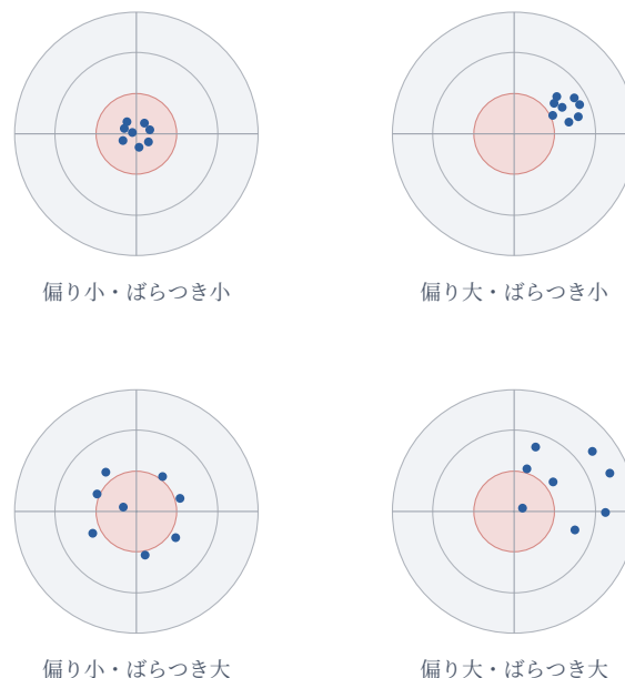
図 9.15 偏りとばらつきを的当てで見る。中心が真の値、点1つが1回ぶんの訓練データから得た予測である。偏りは点の集まりが中心からどれだけずれているか、ばらつきは点どうしがどれだけ散らばっているかにあたる。右上は毎回同じ答えを出すのを外し、左下は平均すれば中心に来るが1回ごとには大きく外れる。
