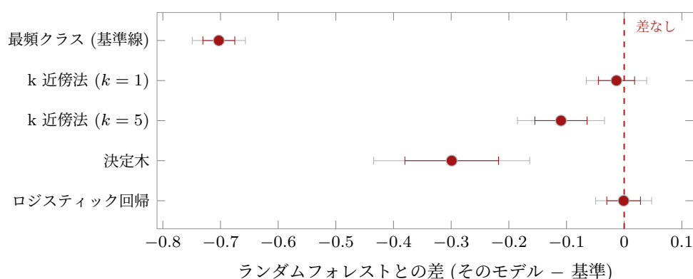
図 8.8 ランダムフォレストを基準にした、層別 5 分割交差検証の平均正解率の差の区間。薄い太い棒は対応を取らずに計算した差の区間、濃い細い棒は同じ分割のフォールドごとに差を取って計算した区間である。赤い縦線が「差なし」で、区間がこの線をまたいでいれば差があるとは言えない。重なりを目で測る余地がない。区間は図 8.7 と同じくフォールド間の SD/\sqrt{5} から作った目安で、正式な 95% の被覆は保証しない。
