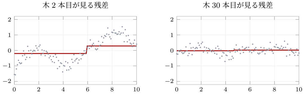
図 7.11 残差 (灰色の点) と、それに当てはめた決定株 (赤)。回を追うごとに残差が小さくなり、木の刻み幅も細くなる。
