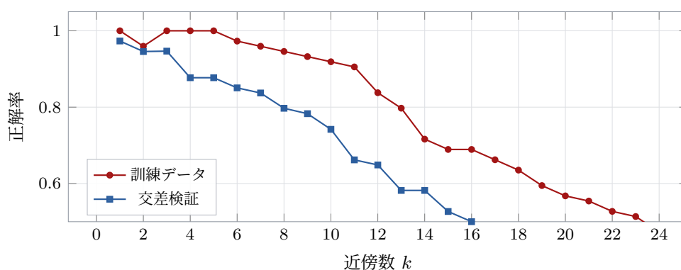
図 8.14 k 近傍法の近傍数 k と正解率。 k が小さいほど複雑なモデルになる。
