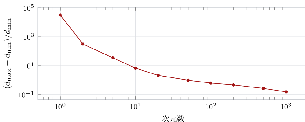
図 4.18 次元と距離の相対的な広がり。次元が上がるほど、最も近い点と最も遠い点の差が消えていく。
