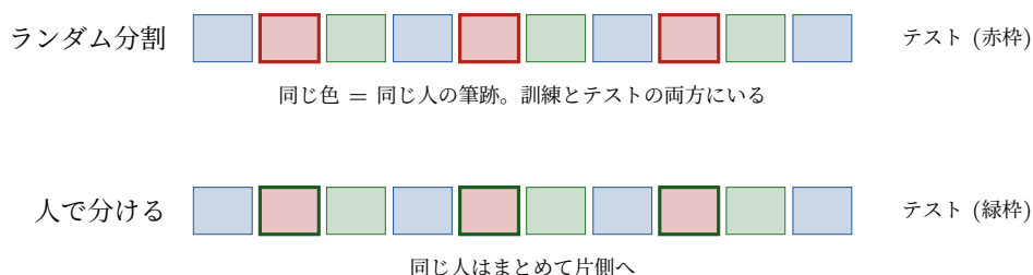
図 9.6 文字認識でのグループ漏れ。人の筆跡の癖を覚えれば当たってしまう。
