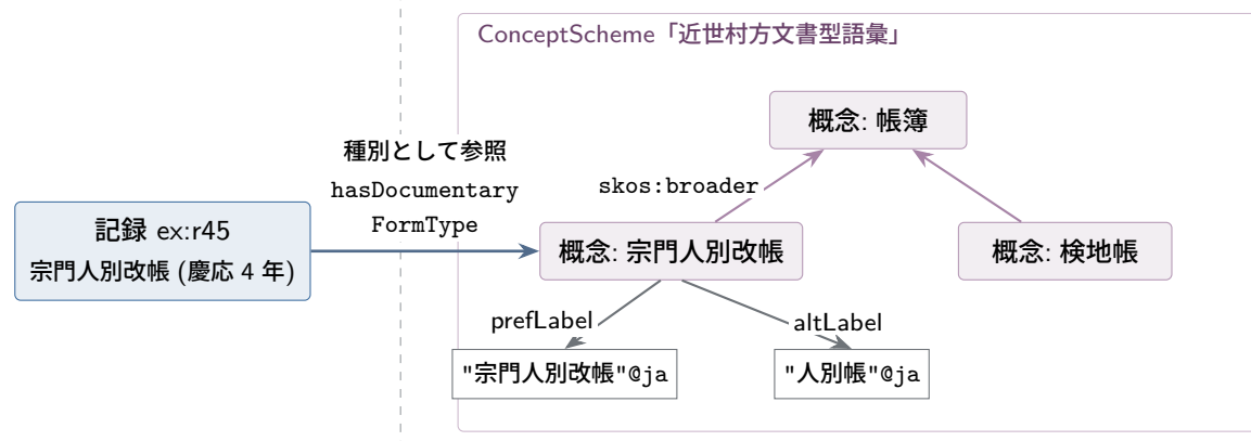
図 7.5 SKOS 語彙の構造。概念は IRI を持つ個体で、ラベル ( prefLabel / altLabel ) と概念間の上下 ( broader ) を持ち、語彙全体は ConceptScheme にまとまる。データの側は種別として概念を参照するだけでよく、表記ゆれは語彙側が吸収する。
