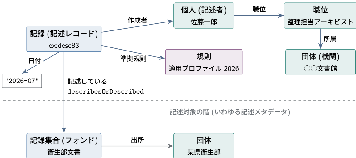
図 4.11 記述の記述の仕組み。目録データそのもの (記述レコード) が一段上の階の記録になり、記述者・規則・日付はその属性・関係として付く。2つの階は rico:describesOrDescribed という通常の関係でつながる。記述者・職位・機関は、記述対象の階の実体とまったく同じクラスである。
