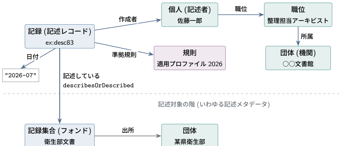
図 4.11 記述の記述の仕組み。目録データそのもの (記述レコード) が一段上の階の記録になり、記述者・規則・日付はその属性・関係として付く。2つの階は rico:describesOrDescribed という通常の関係でつながる。記述者・職位・機関は、記述対象の階の実体とまったく同じクラスである。
