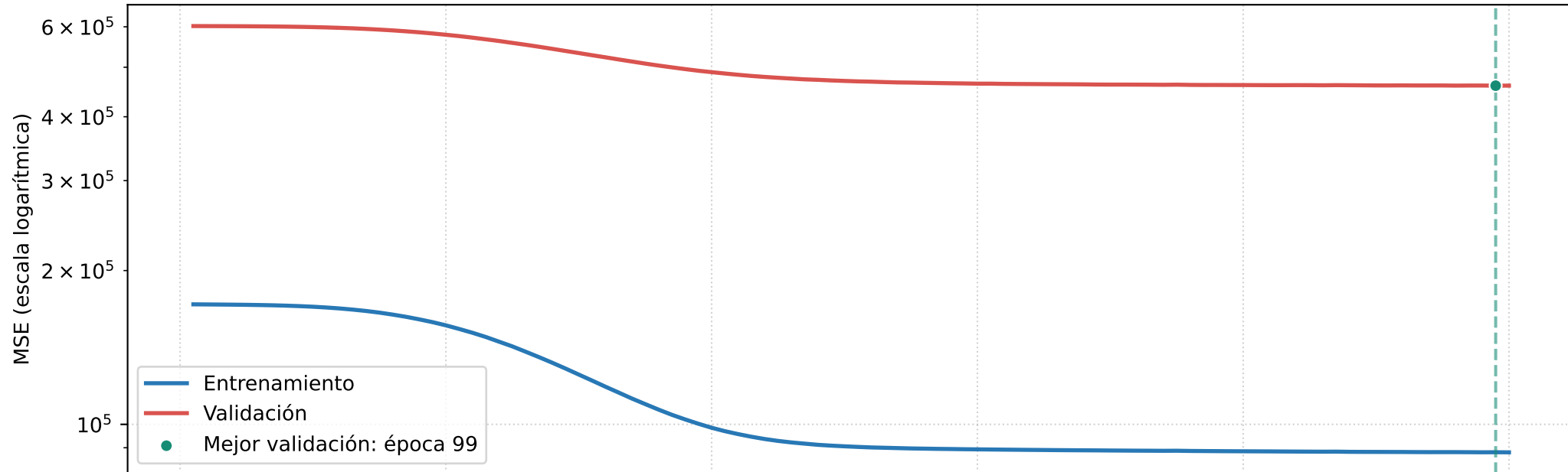
Pérdida por época: menor suele ser mejor
