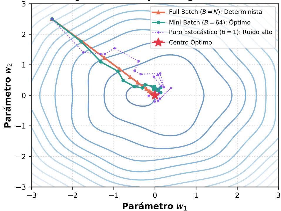
Navegación en el Espacio según Batch Size
