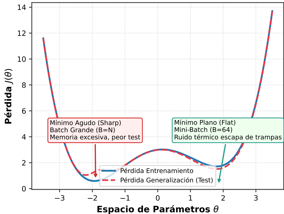
Geometría del Espacio: Mínimos Agudos vs Planos
