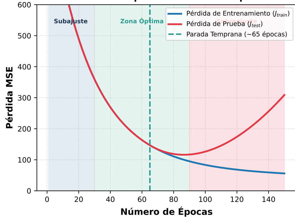
Dinámica Temporal de Pérdida vs Épocas
