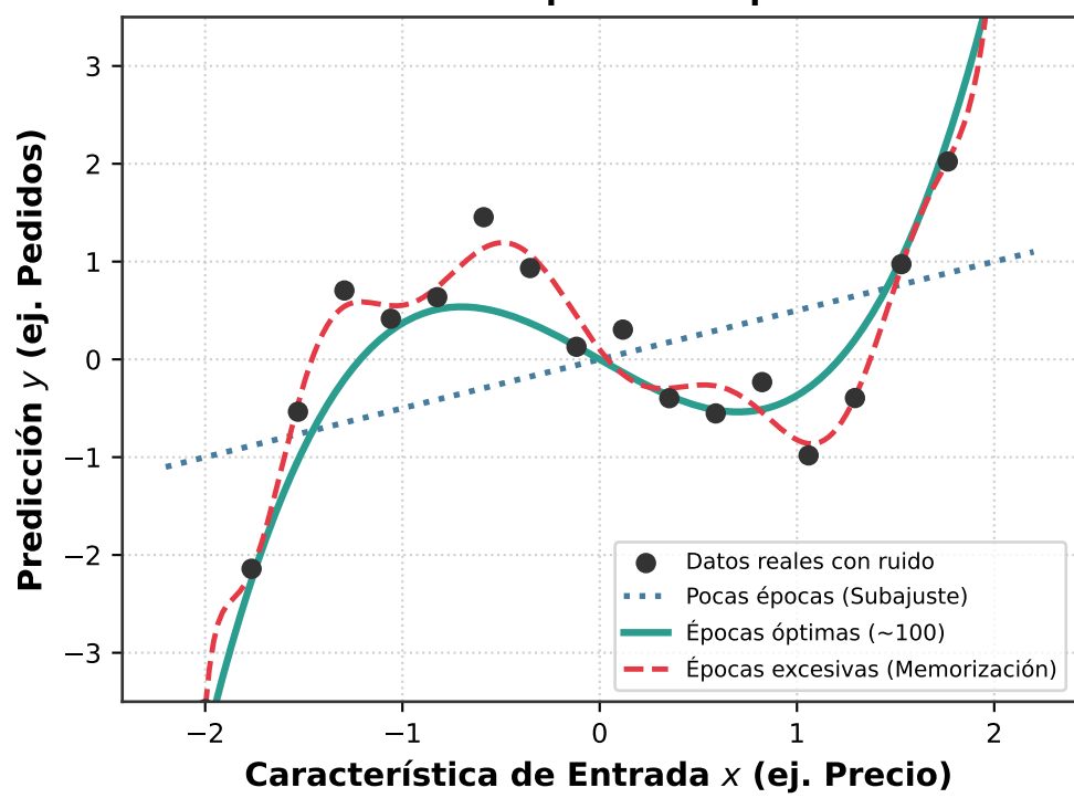
Efecto en el Espacio de Hipótesis \mathcal{H}
