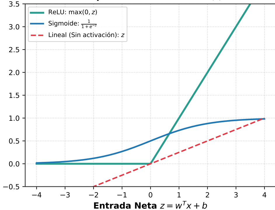
Respuestas de Activación \sigma(z)
