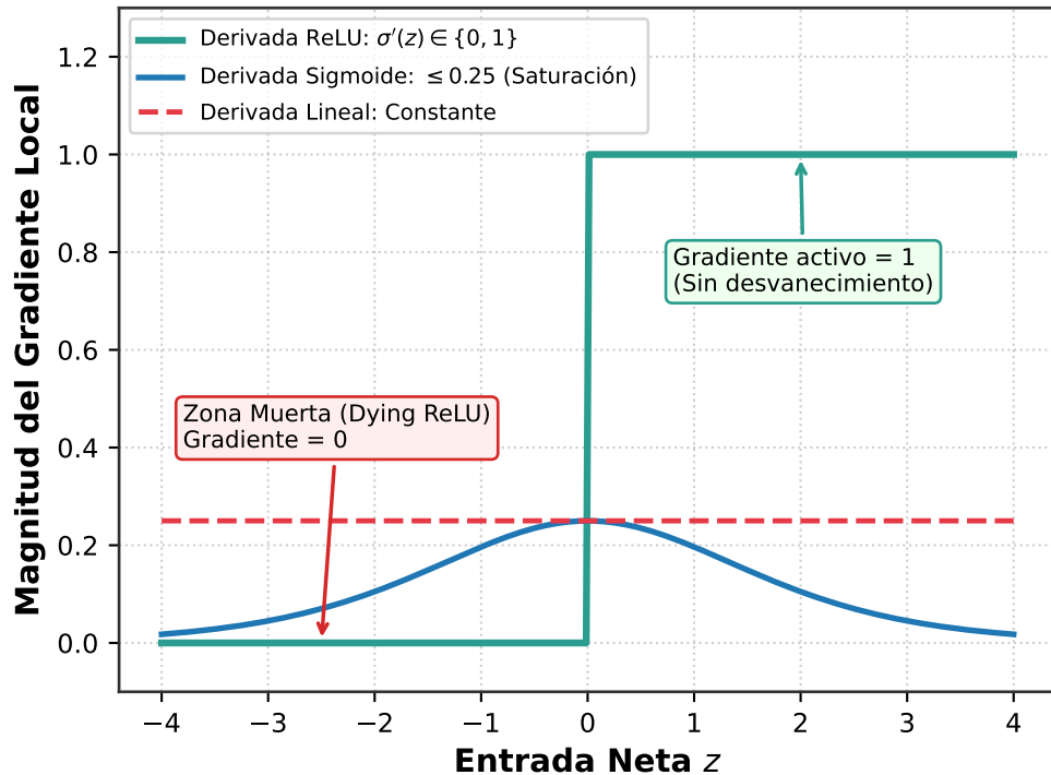
Derivada del Gradiente \sigma'(z) (Propagación)
