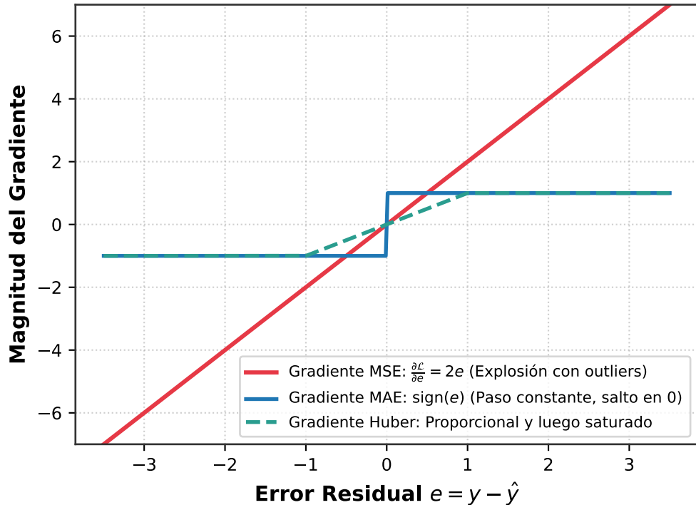
Gradiente Local \partial \mathcal{L} / \partial e (Fuerza de Actualización)
