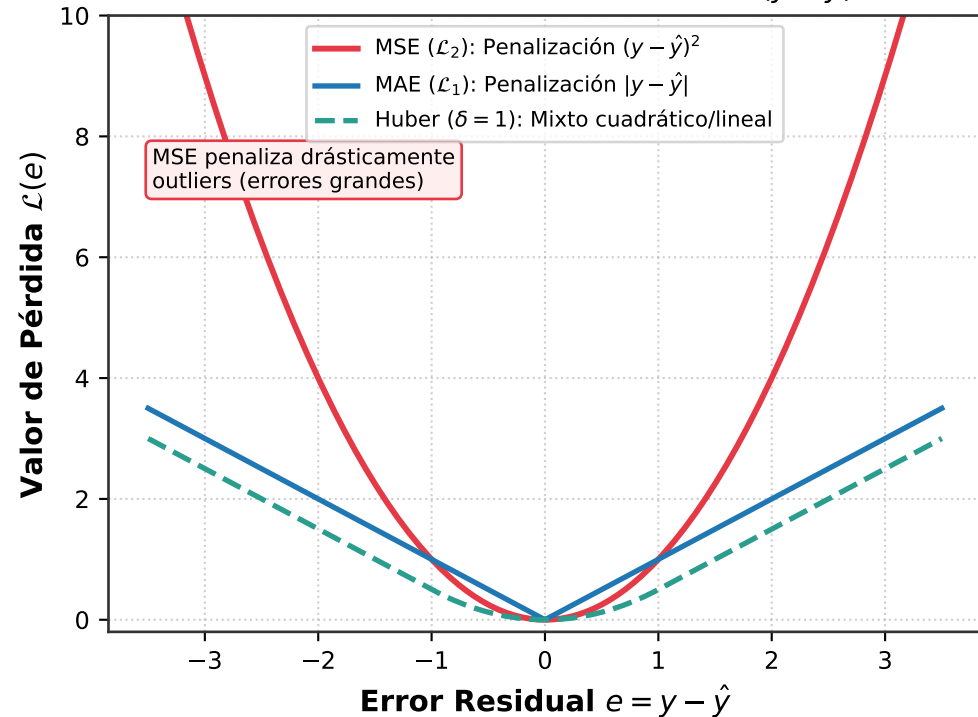
Penalización del Error Residual ( y - \hat{y} )
