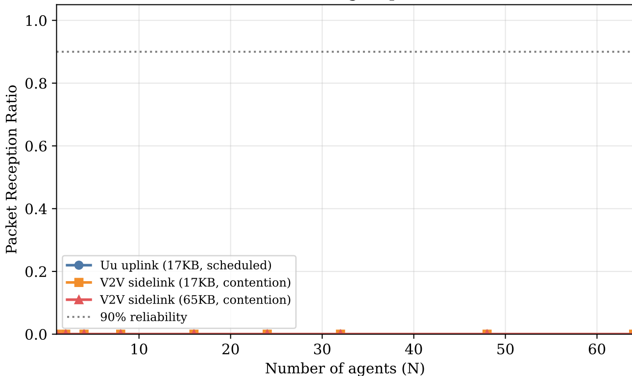
ns-3 5G-LENA NR V2X: Edge Uplink vs V2V Sidelink
