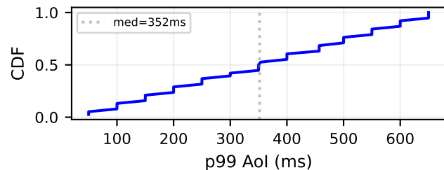
Oracle+SBA
