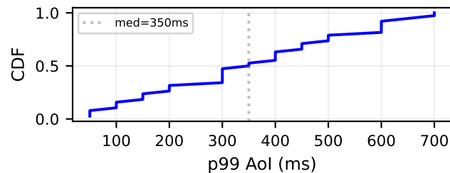
VIPS+SBA
