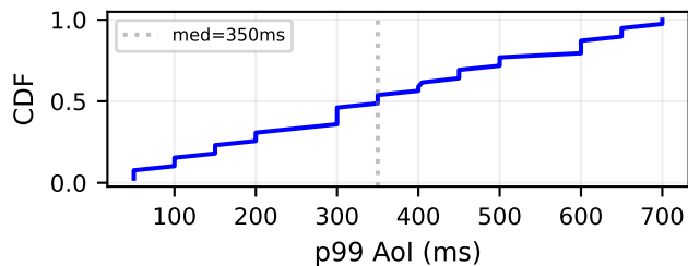
VIPS
