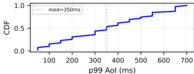
Oracle
