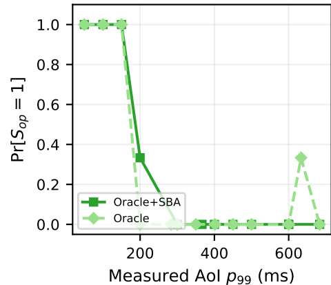
Oracle
