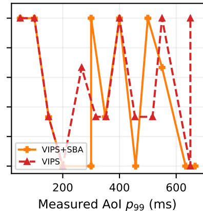
VIPS
