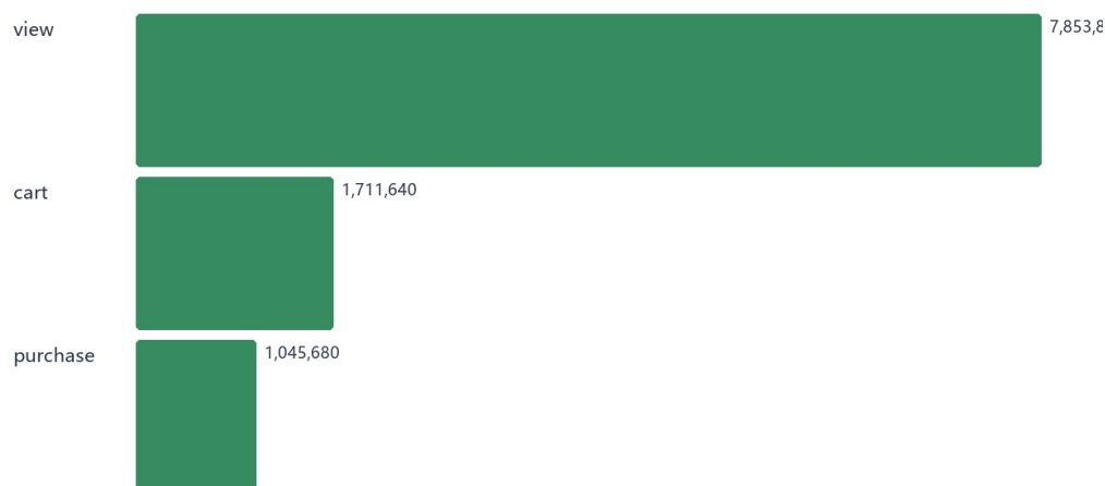
转化漏斗估计用户规模
