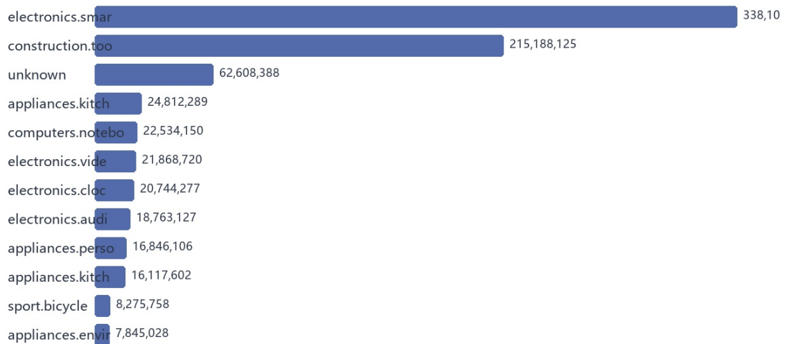
销售额最高的品类 Top 12
