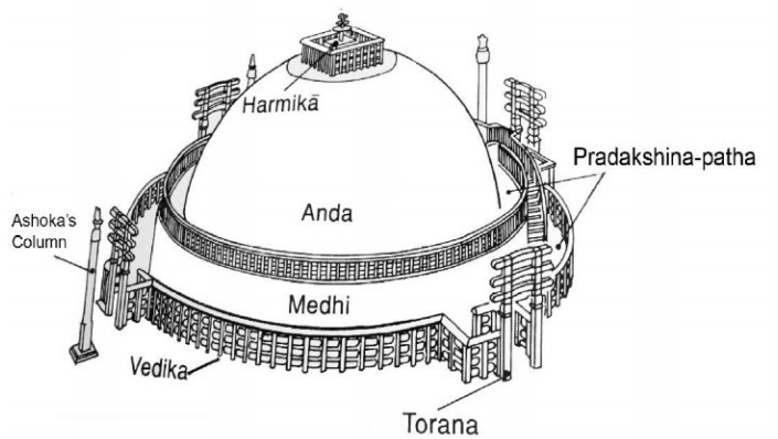
చిత్రం 20.15: అమరావతి స్థూప పునర్నిర్మాణ నమూనా
