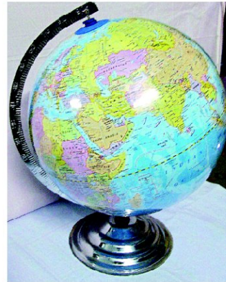
చిత్రం 2.2: గ్లోబు
