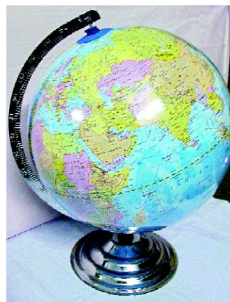
Fig. 2.2: A Globe
