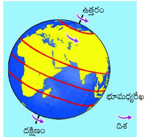
చిత్రం 2.3: భ్రమణాక్షం
