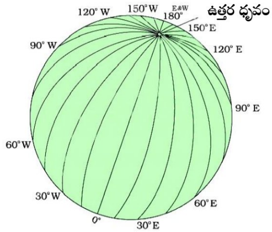
చిత్రం 2.5: గ్లోబుపై రేఖాంశాలు
