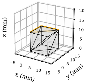
(d) inconsistent winding 3 inconsistent
